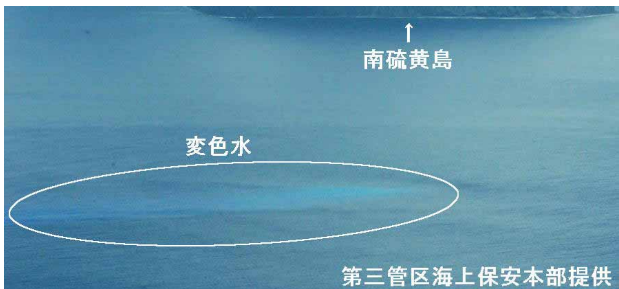
図 3 福德岡ノ場 変色水の状況（27 日、北東側から撮影）
