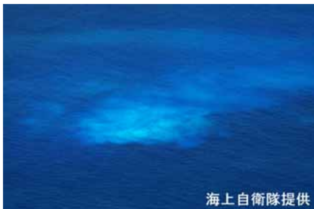
図 1 福德岡ノ場 変色水の状況 （25 日、西側から撮影）
