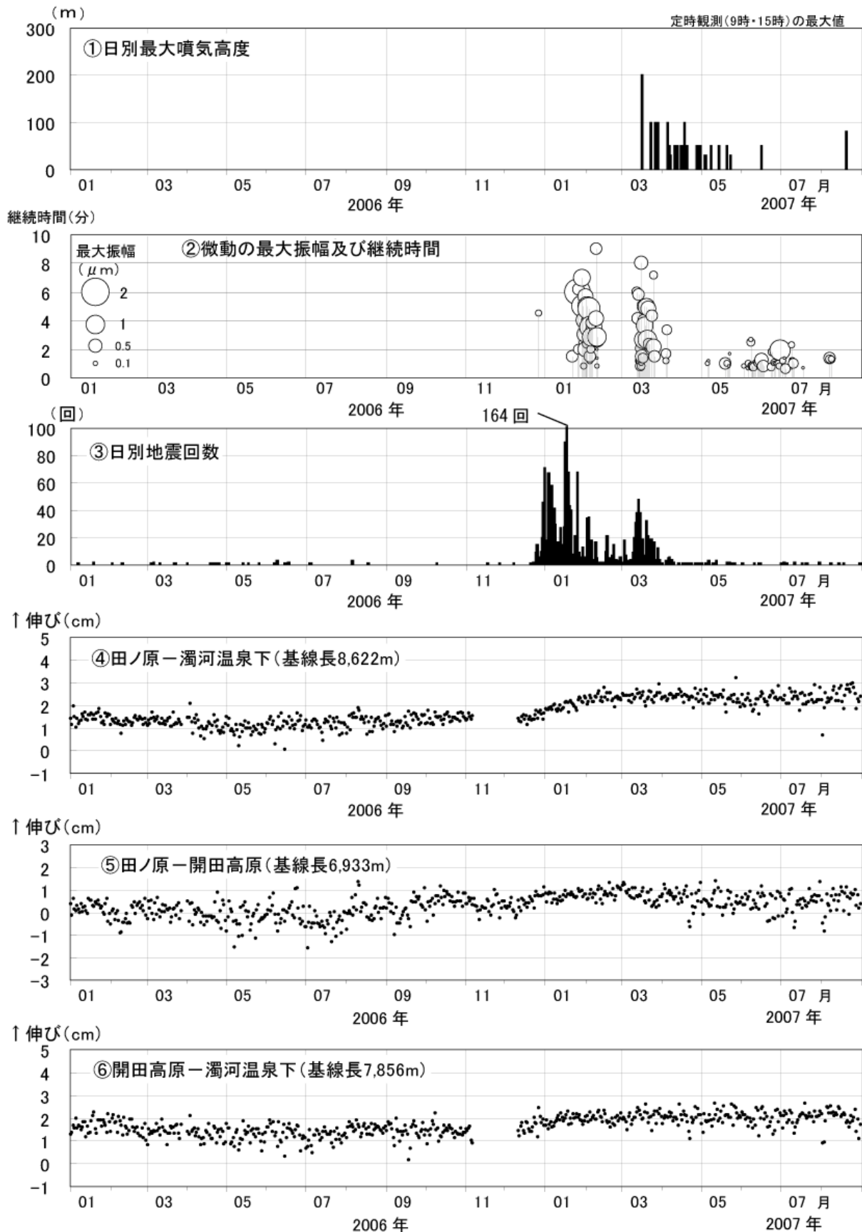
図2 御嶽山 最近の火山活動の推移(2006年1月1日～2007年8月31日)
