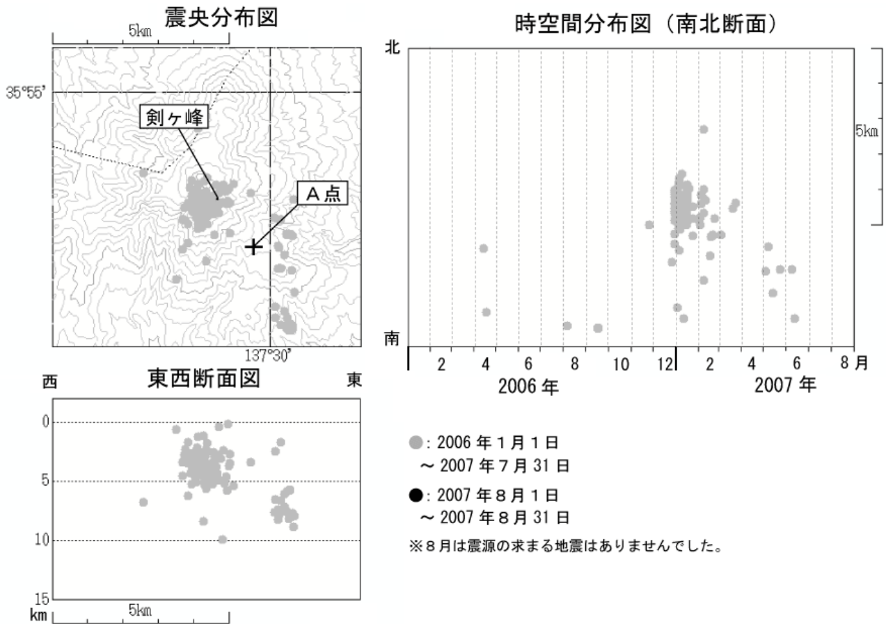
図 3 ※ 御嶽山 山頂付近の地震活動（2006 年 1 月 1 日～2007 年 8 月 31 日） +印は気象庁地震観測点（A点）の位置を示しています。
