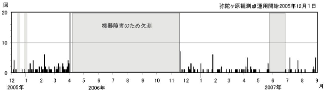
図1 白山 日別地震回数 (2005年12月1日~2007年8月31日)
