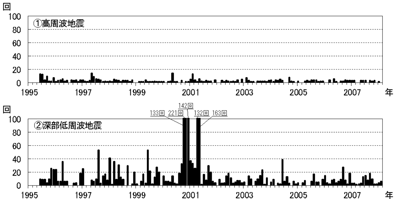
図 1 富士山 月別地震回数(1995 年 6 月～2008 年 2 月)
