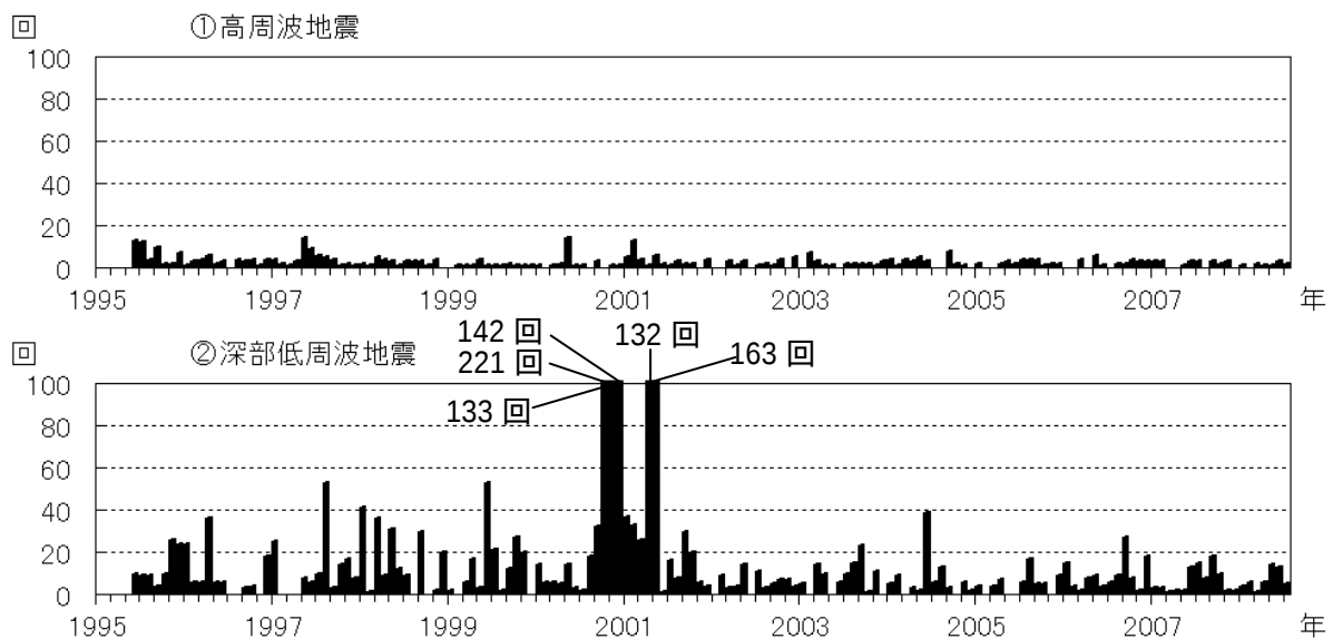
図 1 富士山 月別地震回数(1995 年 6 月～2008 年 7 月)
