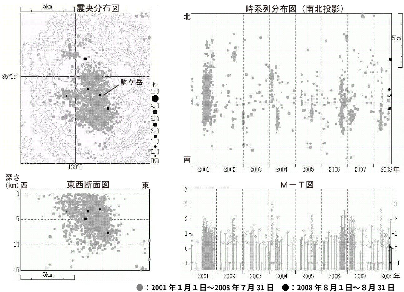
図 3 ※ 箱根山 地震活動経過（2001 年 1 月 1 日～2008 年 8 月 31 日）
