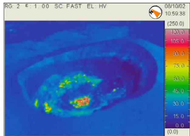
図 4 浅間山 赤外熱映像装置により南西側上空から撮影した山頂火口内の表面温度分布
