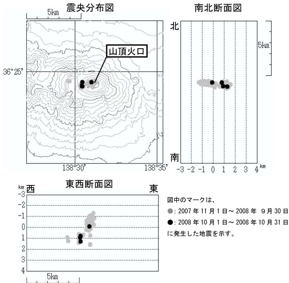
図 5 浅間山 震源分布図（2007 年 11 月 1 日～2008 年 10 月 31 日）
