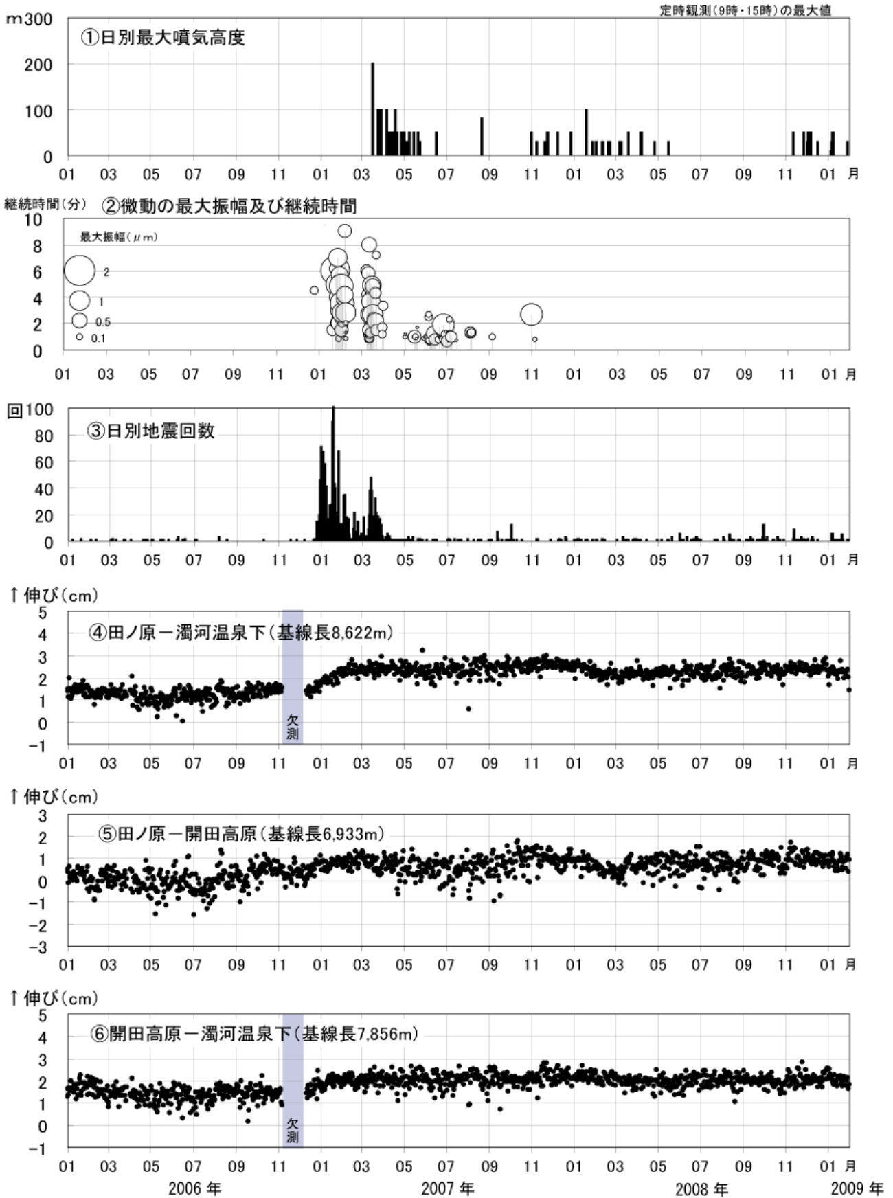
図2 御嶽山 最近の火山活動の推移(2006年1月1日～2009年1月31日)
