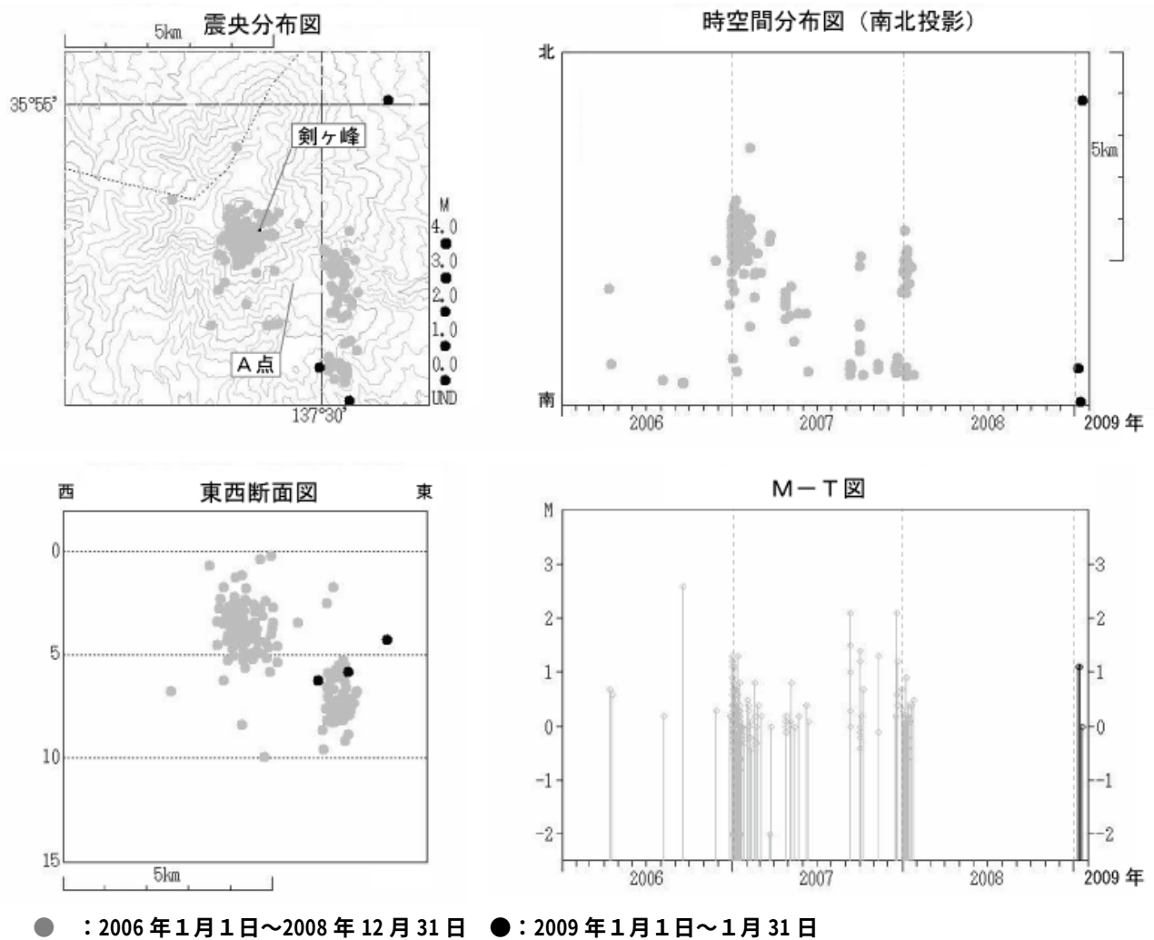
図 4 ※ 御嶽山 震源分布図（2006 年 1 月 1 日～2009 年 1 月 31 日）
