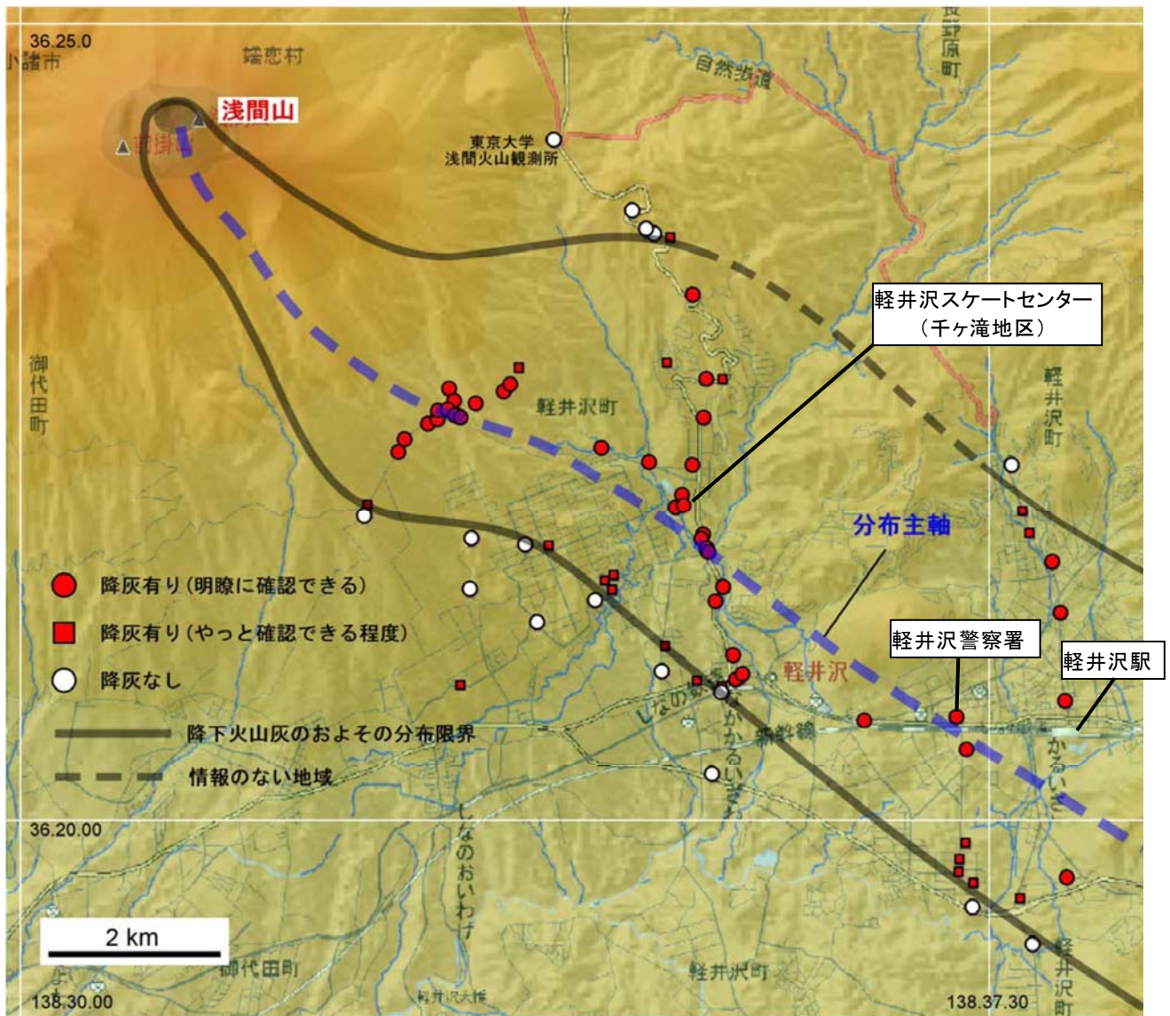
図1 降灰調査実施地点及び降灰分布
