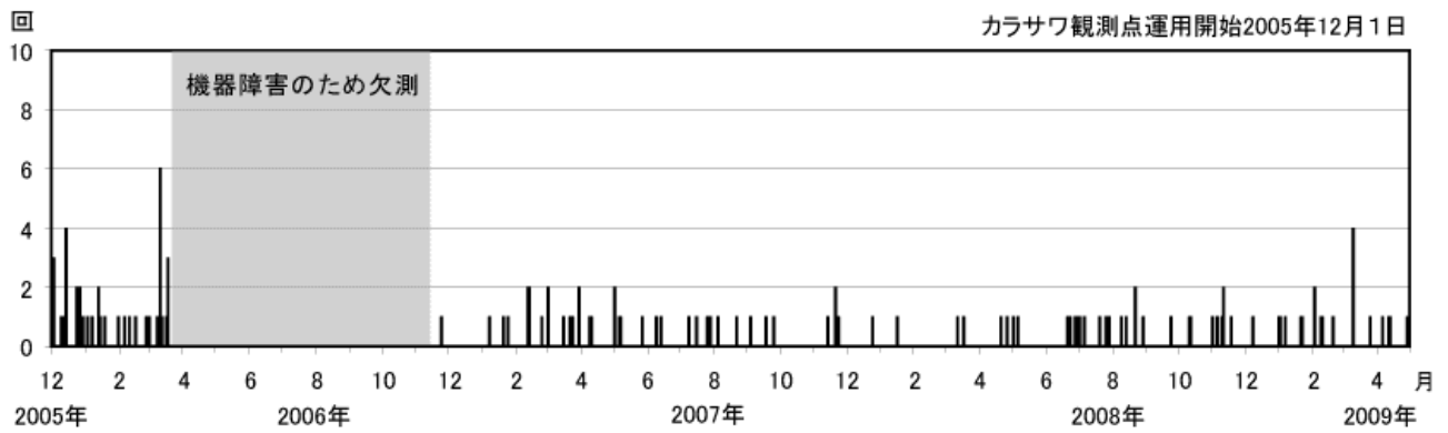
図2 新潟焼山 日別地震回数（2005年12月1日～2009年4月30日）
