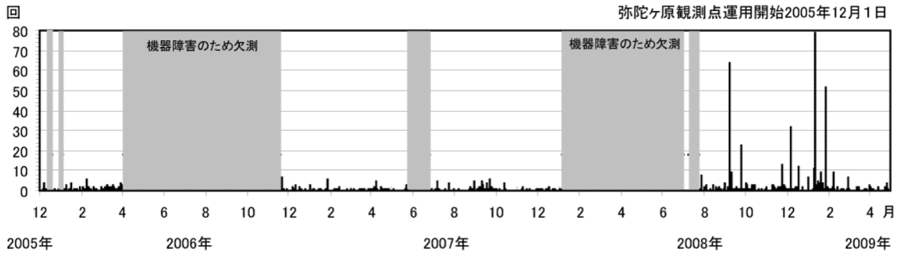
図 2 白山 日別地震回数（2005 年 12 月 1 日～2009 年 4 月 30 日）
