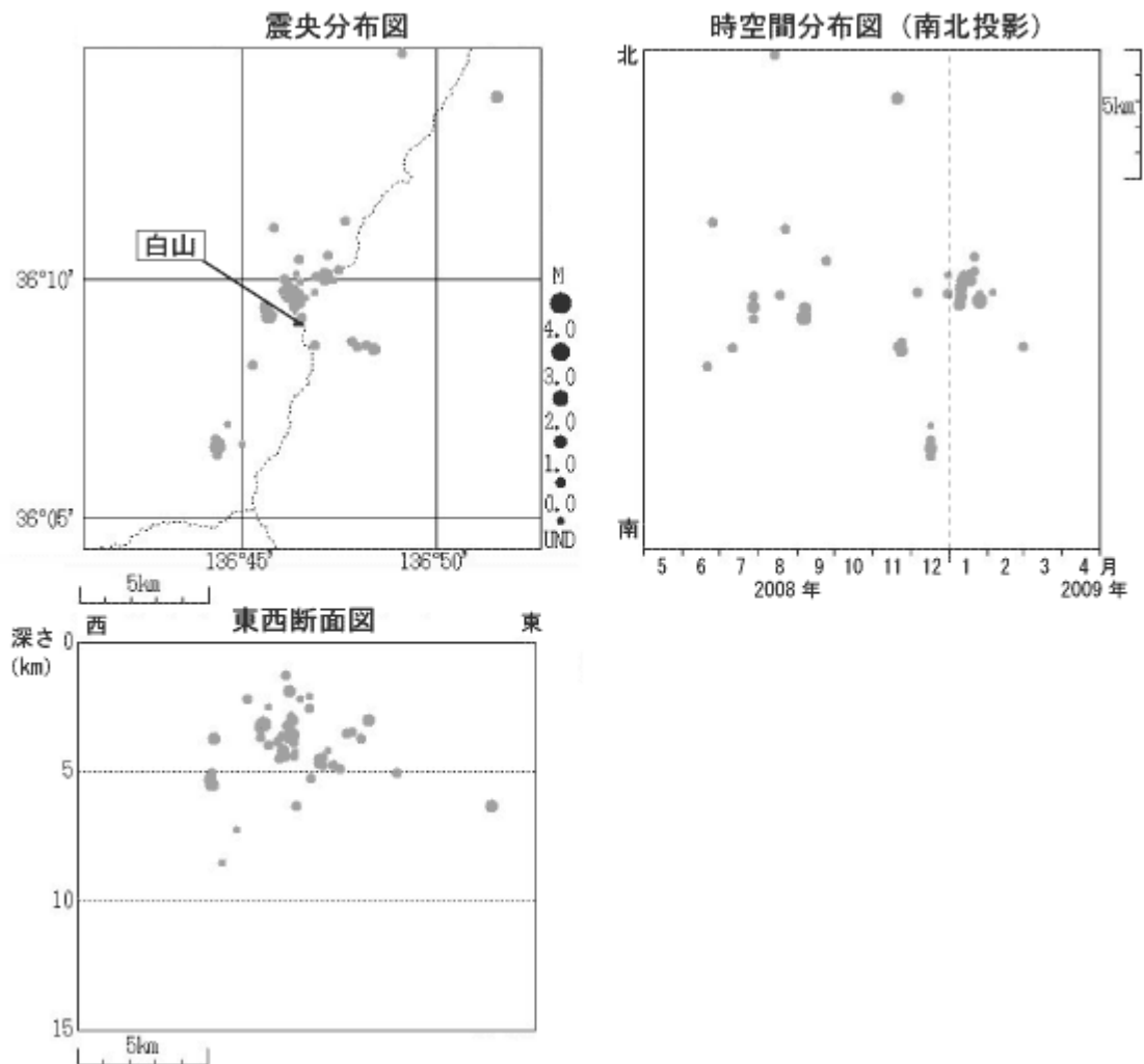
図 3 白山 震源分布図（2008 年 5 月 1 日～2009 年 4 月 30 日）
