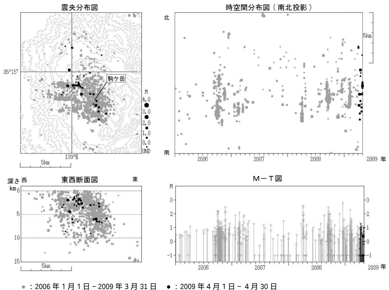
図 3 箱根山 震源分布図（2006 年 1 月 1 日 ~ 2009 年 4 月 30 日） M（マグニチュード）は地震の規模を表します。 図中の震源要素は一部暫定値が含まれており、後日変更することがあります。
