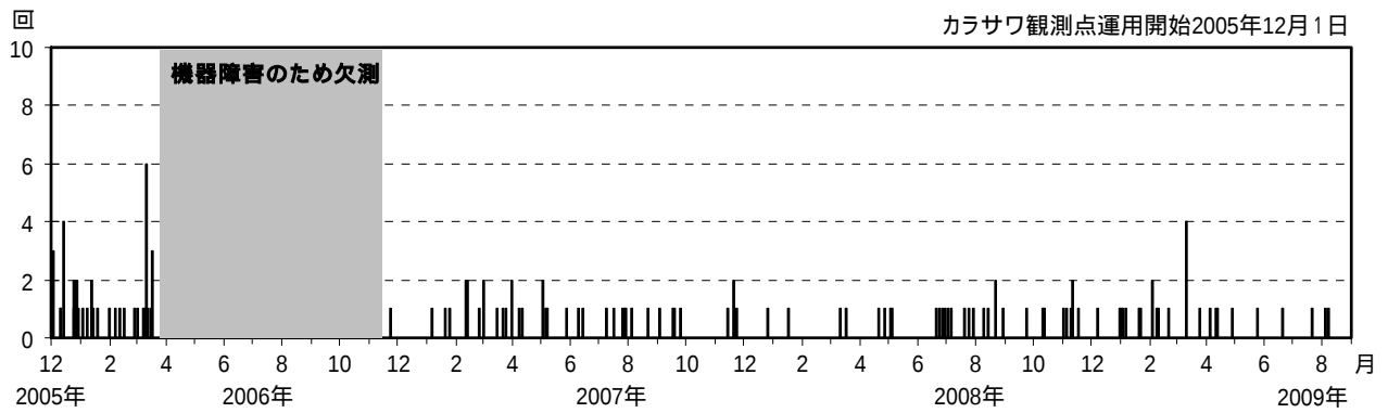
図2 新潟焼山 日別地震回数（2005年12月1日～2009年8月31日）
