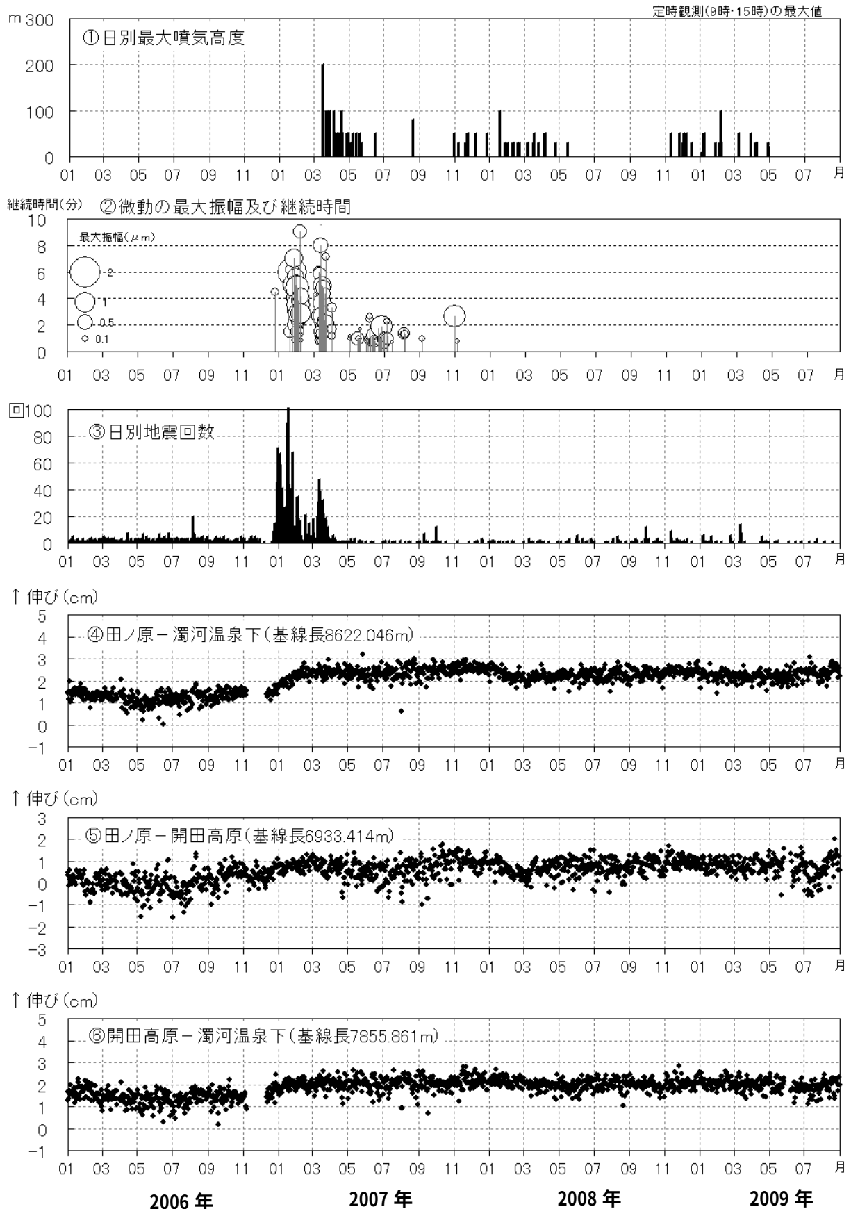
図2 御嶽山 最近の火山活動の推移（2006年1月1日～2009年8月31日）
