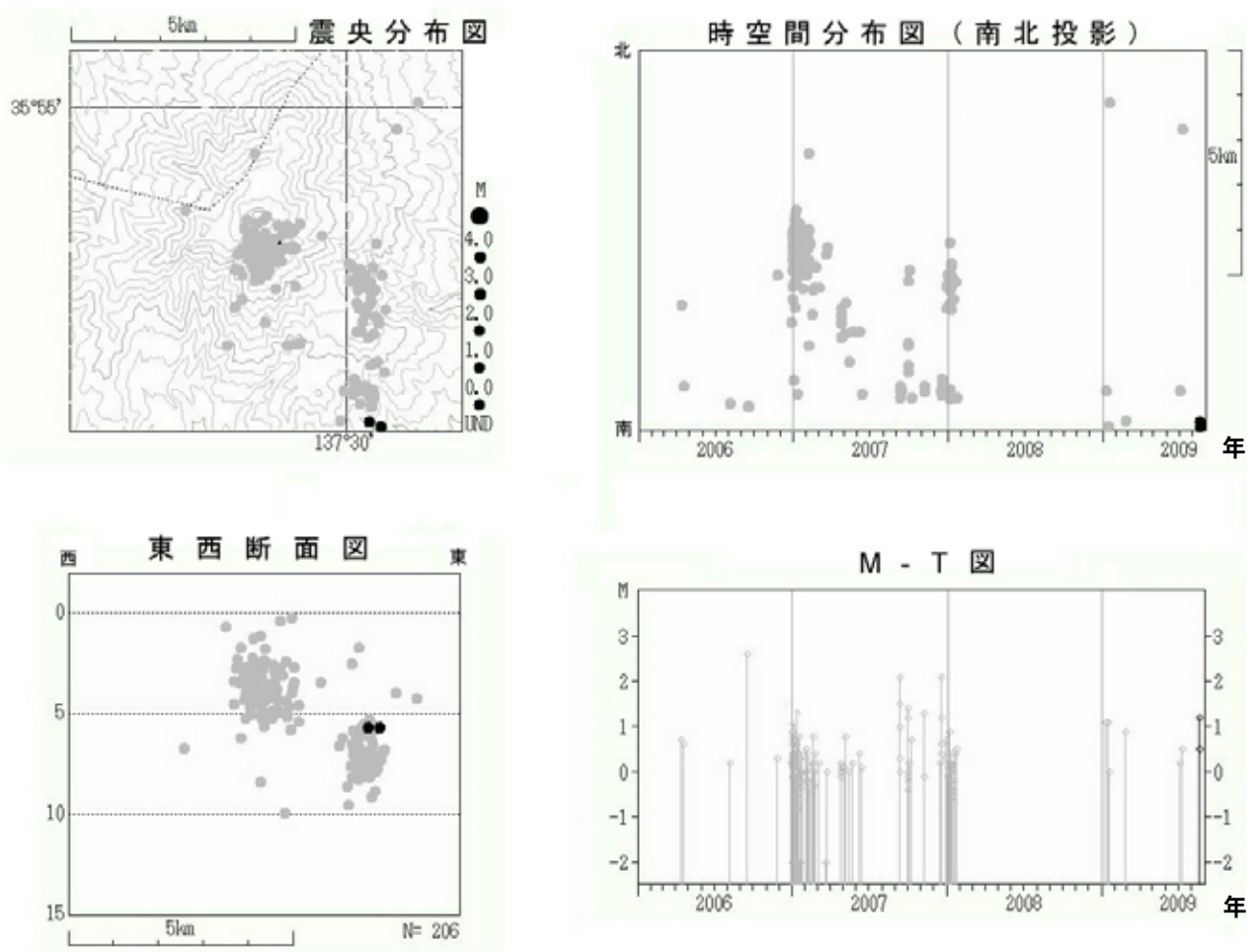
図4※ 御嶽山 震源分布図（2006年1月1日～2009年8月31日）
