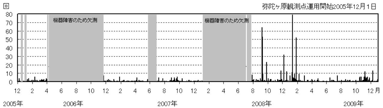
図 2 白山 日別地震回数（2005 年 12 月 1 日～2009 年 12 月 31 日）
