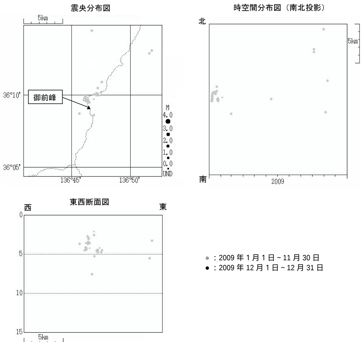
図 3 白山 震源分布図（2009 年 1 月 1 日～12 月 31 日）
