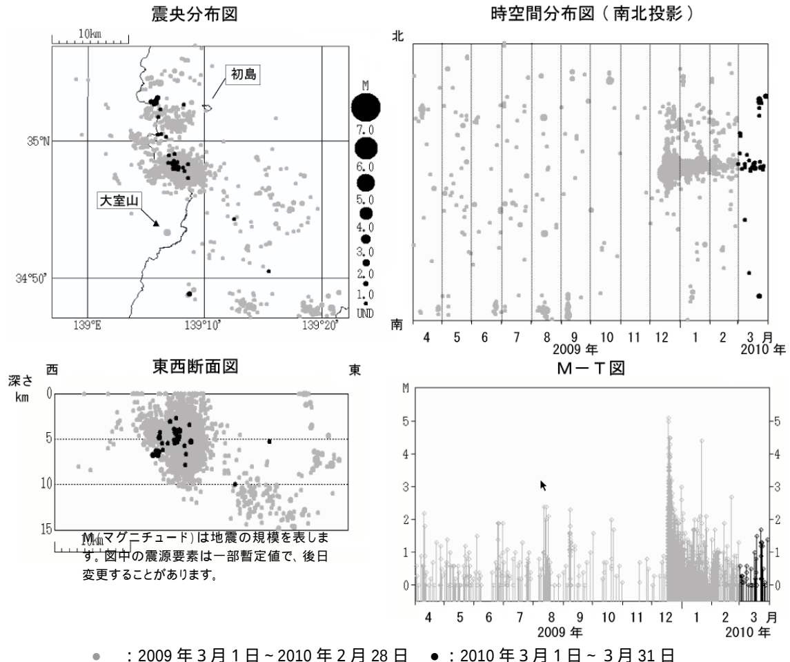
図 1 伊豆東部火山群 震源分布図（2009 年 3 月 1 日～2010 年 3 月 31 日）
