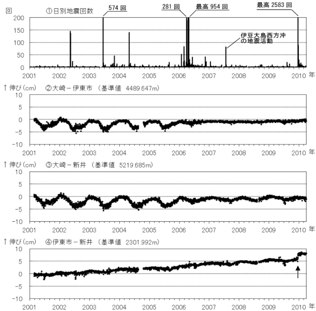
図 2 伊豆東部火山群 最近の火山活動の推移（2001 年 1 月～2010 年 3 月）
