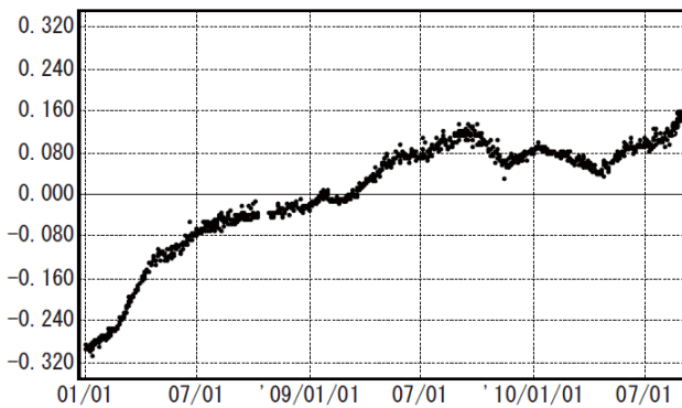
(m) (5) 硫黄島 2 (960605) → M硫黄島 (079073) 南北 基準値：3228.573m
