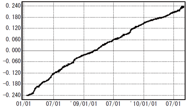
図 1※ 硫黄島 国土地理院による GPS 観測結果 1) (2008 年 1 月 1 日～2010 年 8 月 29 日)
