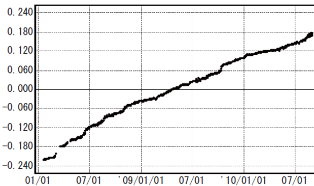
図 1※ 硫黄島 国土地理院による GPS 観測結果 1) (2008 年 1 月 1 日～2010 年 8 月 29 日)
