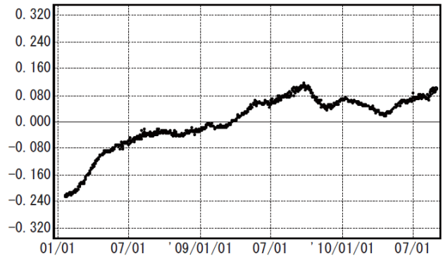
(m) (4) 硫黄島 2 (960605) → 硫黄島 1 (960604) 南北 基準値：3254.910m
