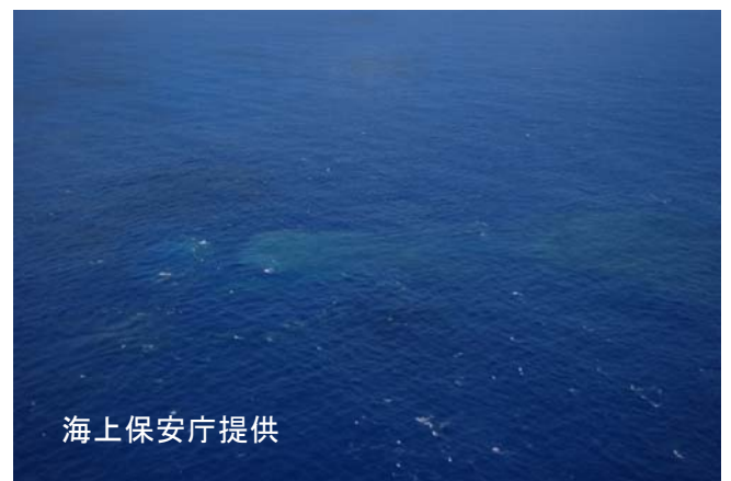
図 2※ 福德岡ノ場 変色水の状況（9 月 29 日撮影）
