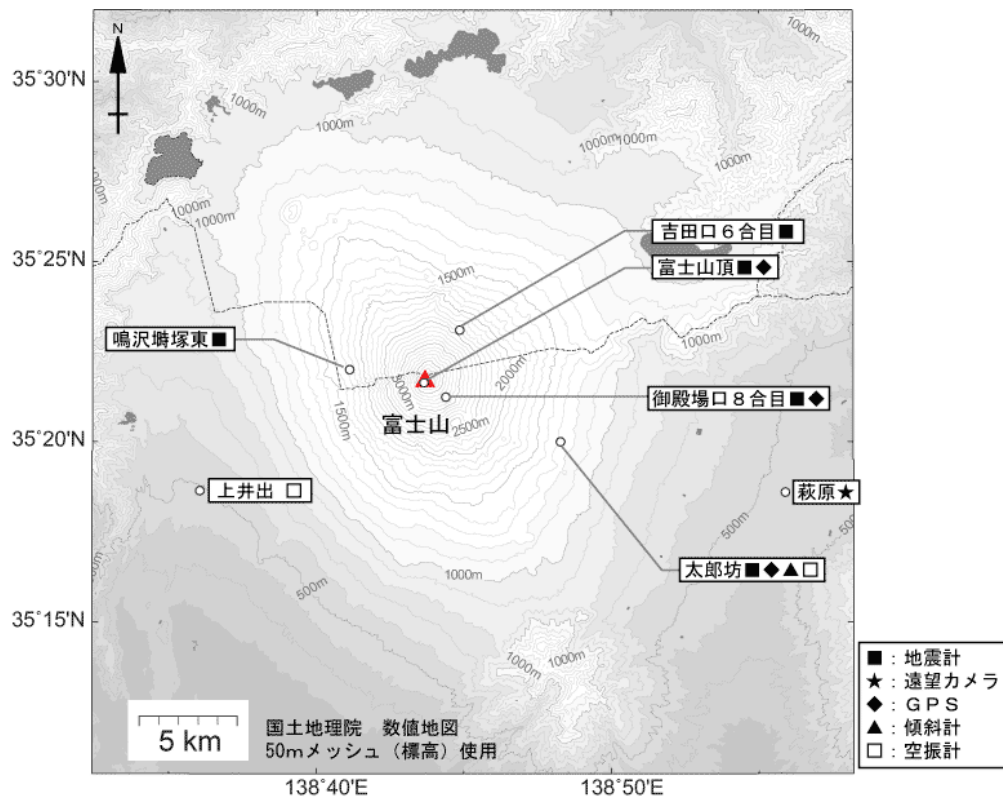
図 4 富士山 気象庁の観測点配置図（小さな白丸は観測点位置を示しています） 運用開始前の観測点も含みます。
