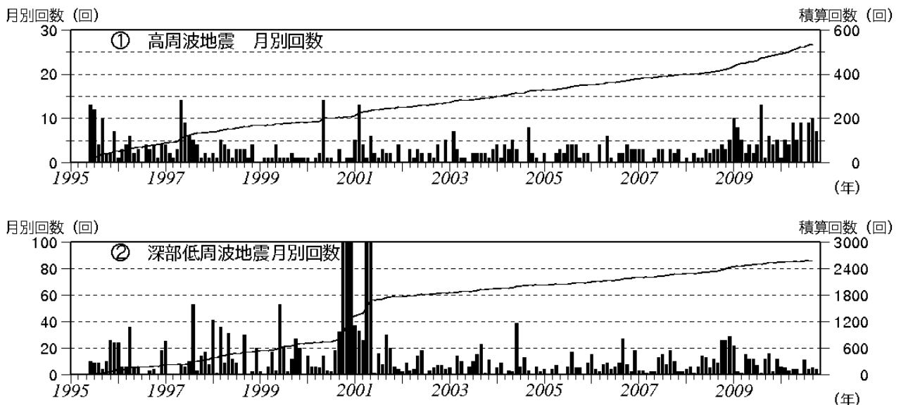
図 1※ 富士山 月別地震回数(1995 年 6 月～2010 年 10 月)
