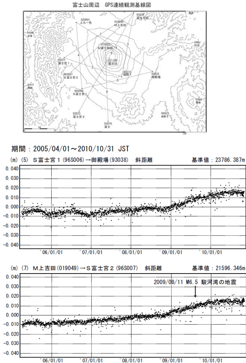
図 3※ 富士山 国土地理院による GPS 観測結果 1) (2005 年 4 月 1 日～2010 年 10 月 31 日)
