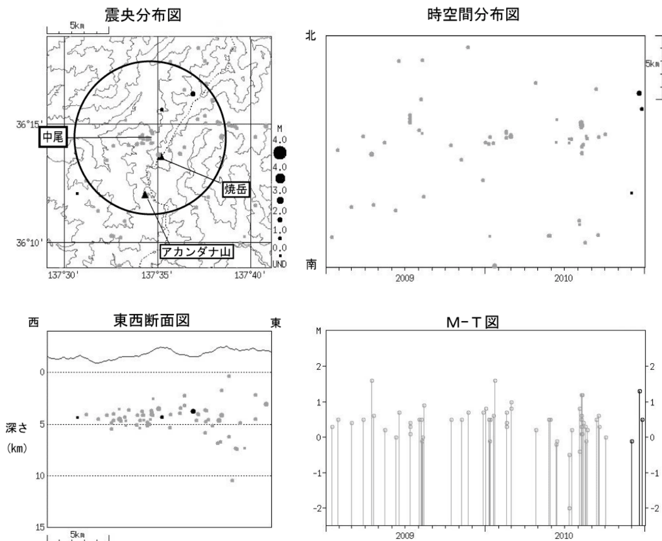
図 3※ 焼岳 広域ネットによる山体・周辺の地震活動(2009 年 1 月 1 日～2010 年 12 月 31 日)
