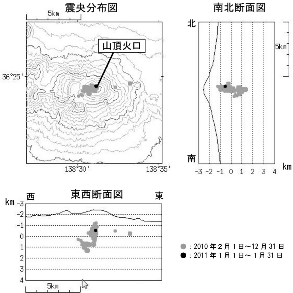
図 4 ※ 浅間山 震源分布図（2010 年 2 月 1 日～2011 年 1 月 31 日）
