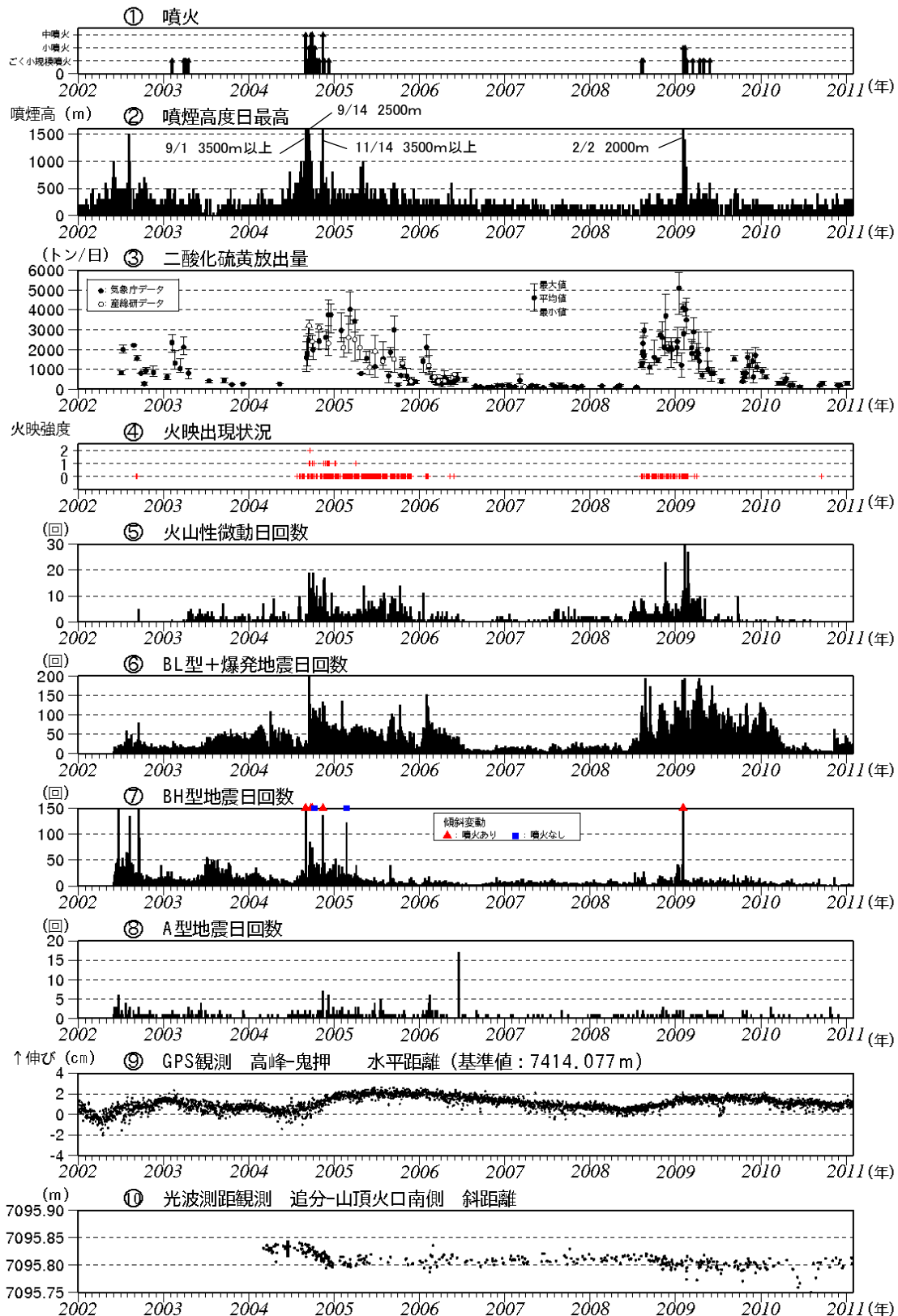
図 3※ 浅間山 最近の火山活動の推移 (2002 年 1 月 1 日～2011 年 1 月 31 日)
