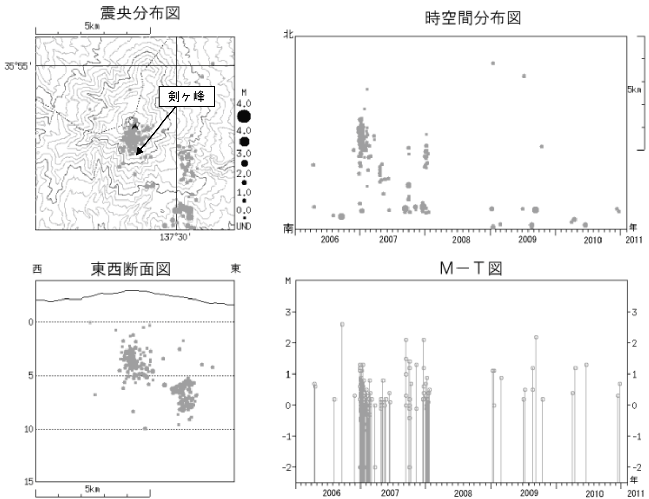
図 4※ 御嶽山 震源分布図（2006 年 1 月 1 日～2011 年 1 月 31 日）
