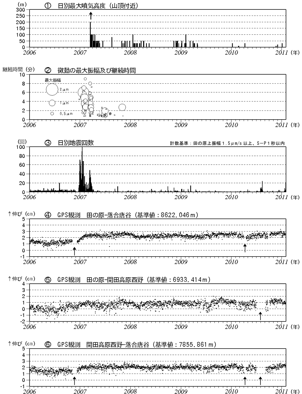
図 3 御嶽山 最近の火山活動の推移（2006 年 1 月 1 日～2011 年 1 月 31 日）
