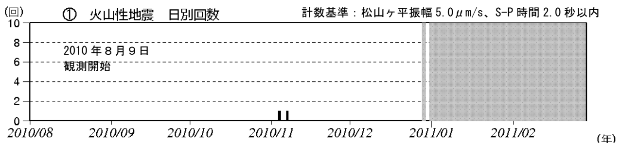
図 3 青ヶ島 火山性地震日別回数（2010 年 8 月 1 日～2011 年 2 月 28 日）
