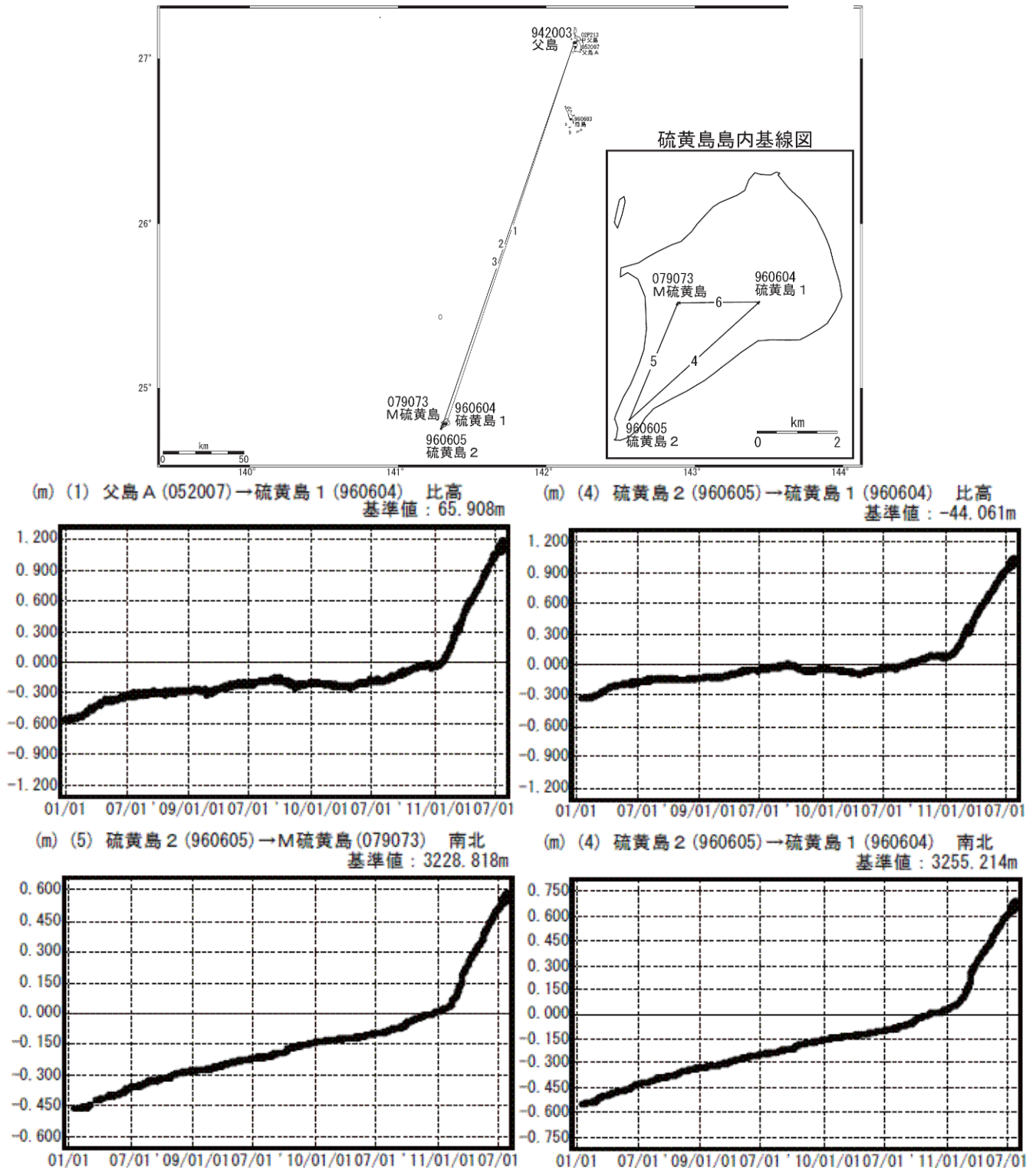
図 3※ 硫黄島 国土地理院による GPS 観測結果 1) (2008 年 1 月 1 日～2011 年 7 月 25 日)
