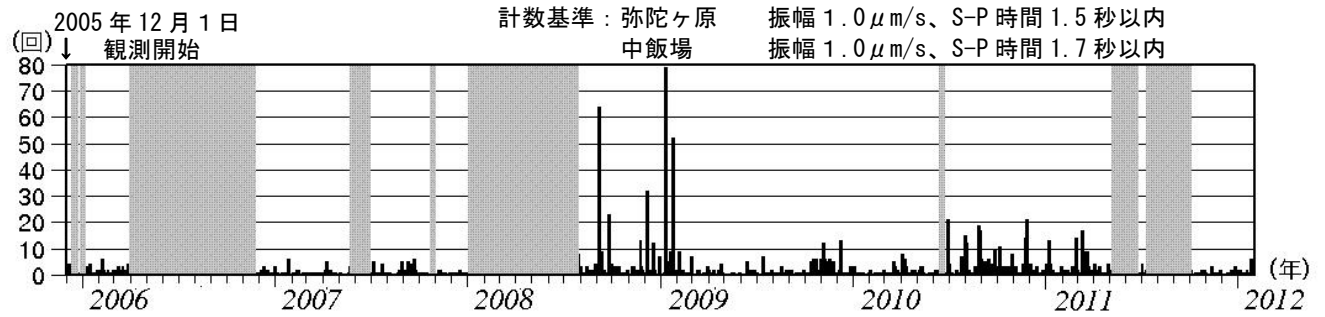
図 3 白山 日別地震回数（2005 年 12 月～2012 年 1 月）
