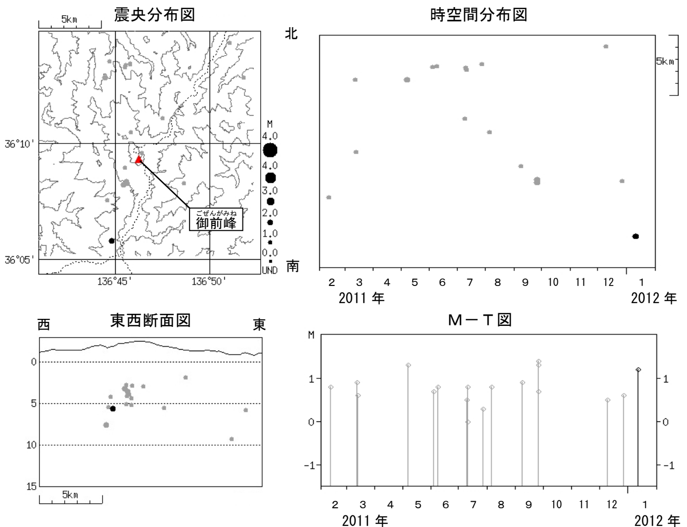
図 4※白山 広域地震観測網による山体・周辺の地震活動（2011 年 2 月～2012 年 1 月）
