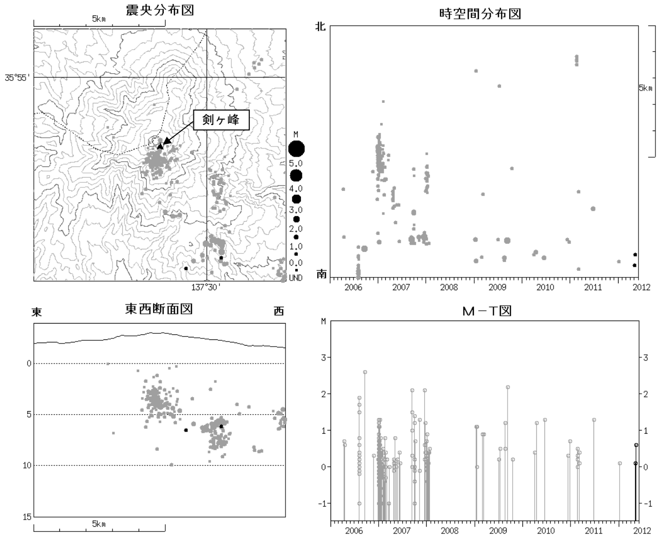
図 4 ※ 御嶽山 広域地震観測網による山体・周辺の震源分布図（2006 年 1 月 1 日～2012 年 5 月 31 日） ●：2006 年 1 月 1 日～2012 年 4 月 30 日 ●：2012 年 5 月 1 日～5 月 31 日 M（マグニチュード）は地震の規模を表します。 図中の震源要素は一部暫定値が含まれており、後日変更することがあります。
