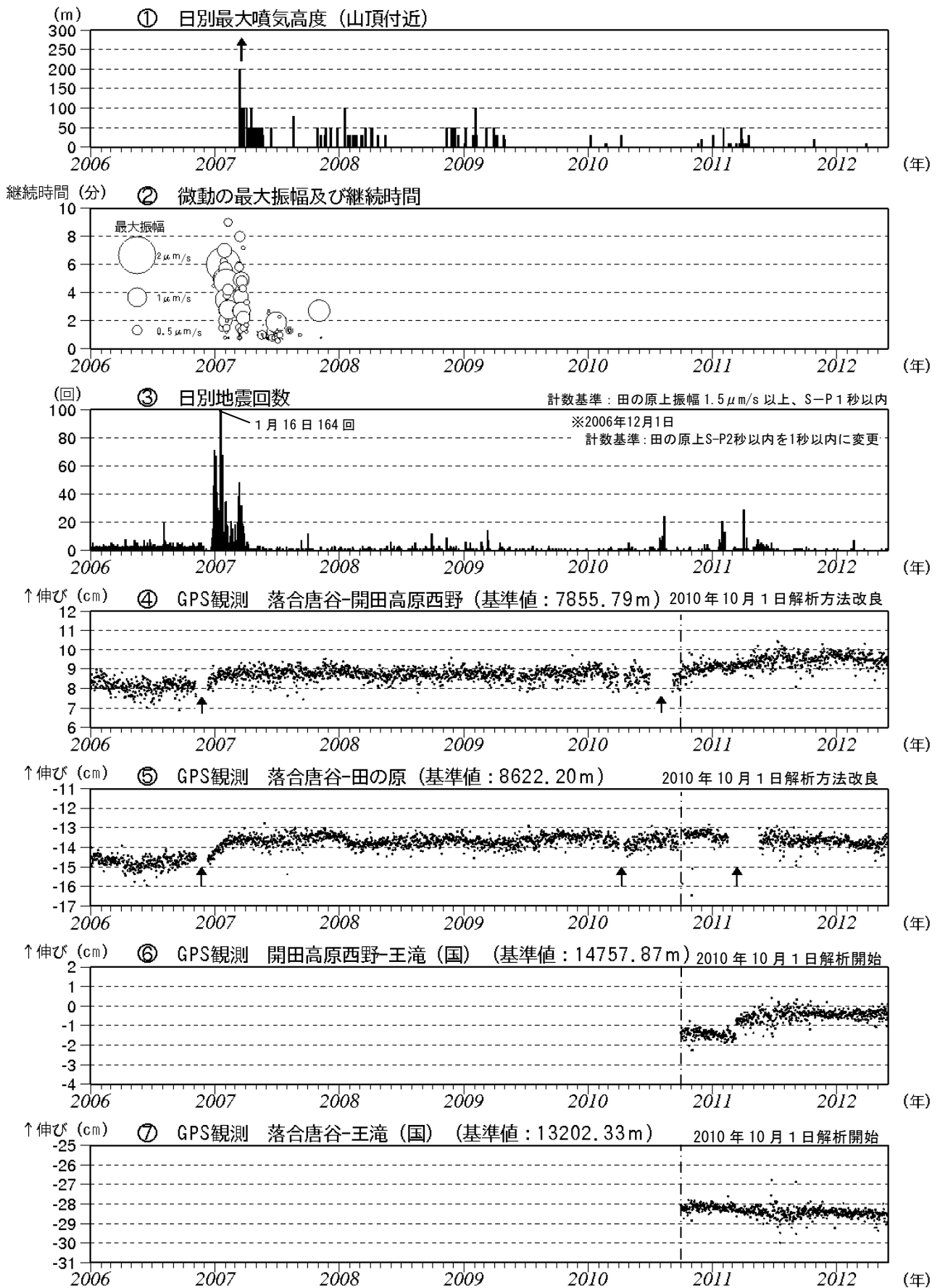
図3 御嶽山 最近の火山活動経過図（2006年1月1日～2012年5月31日）
