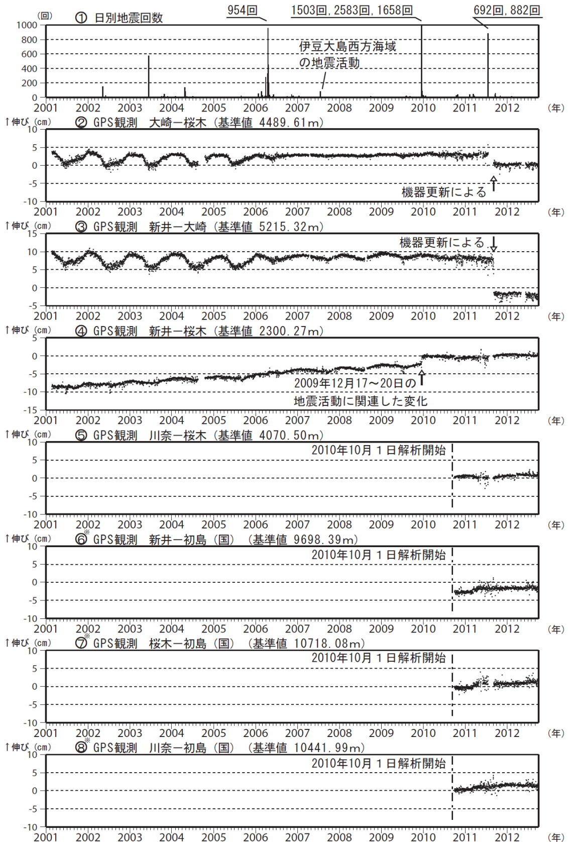
図3 伊豆東部火山群 最近の火山活動経過図（2001年1月～2012年9月）
