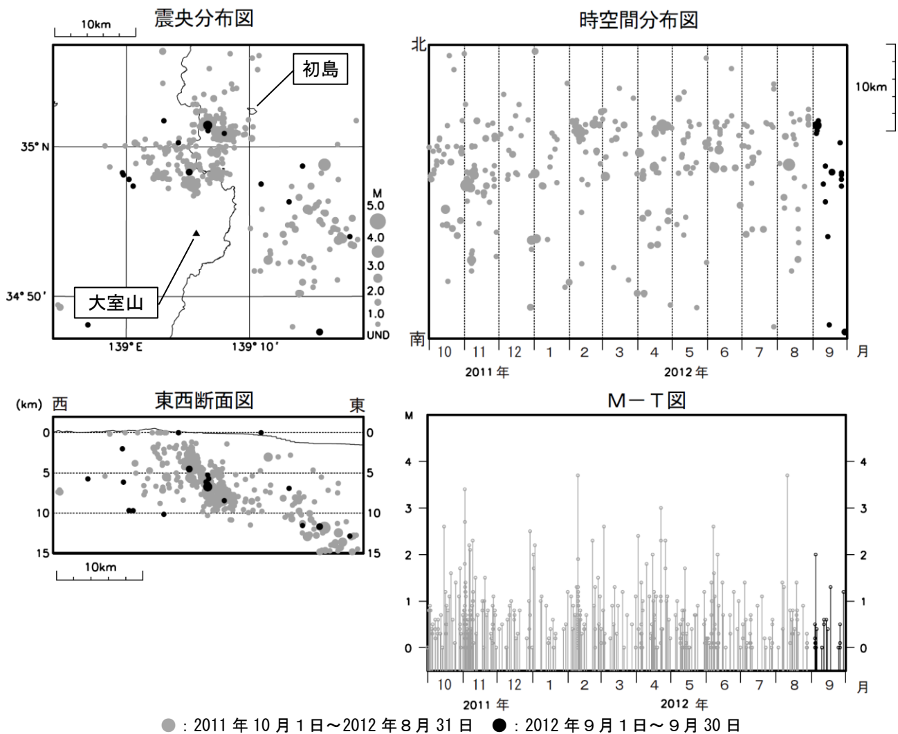
図 2※ 伊豆東部火山群 広域地震観測網による震源分布図（2011 年 10 月 1 日～2012 年 9 月 30 日） M（マグニチュード）は地震の規模を表します。 図中の震源要素は一部暫定値が含まれており、後日変更することがあります。
