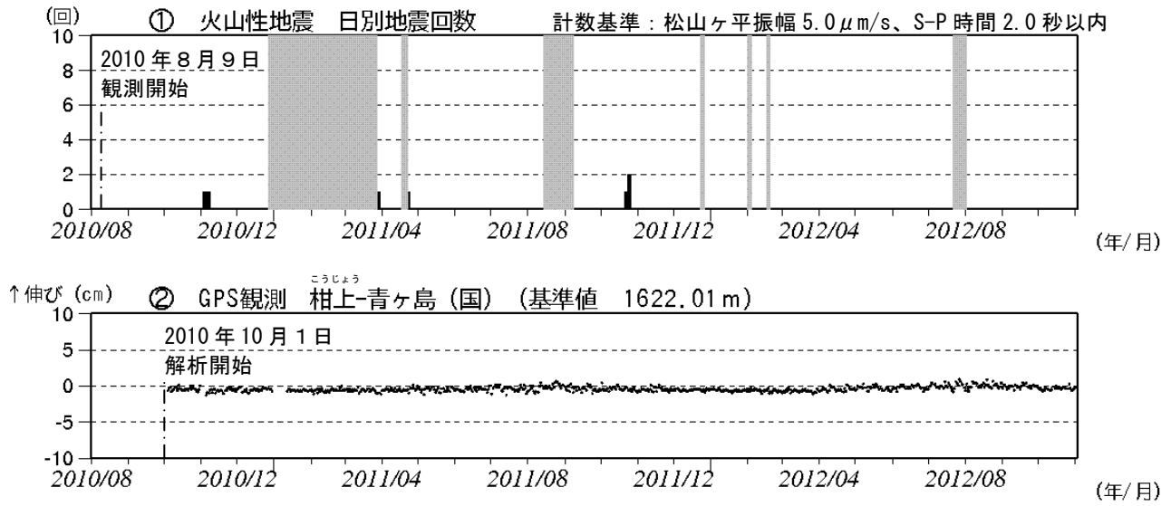
図 2 青ヶ島 火山活動の推移（2010 年 8 月 9 日～2012 年 10 月 31 日）
