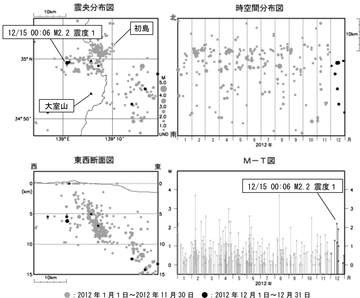
図 2※ 伊豆東部火山群 広域地震観測網による震源分布図（2012 年 1 月 1 日～2012 年 12 月 31 日）
