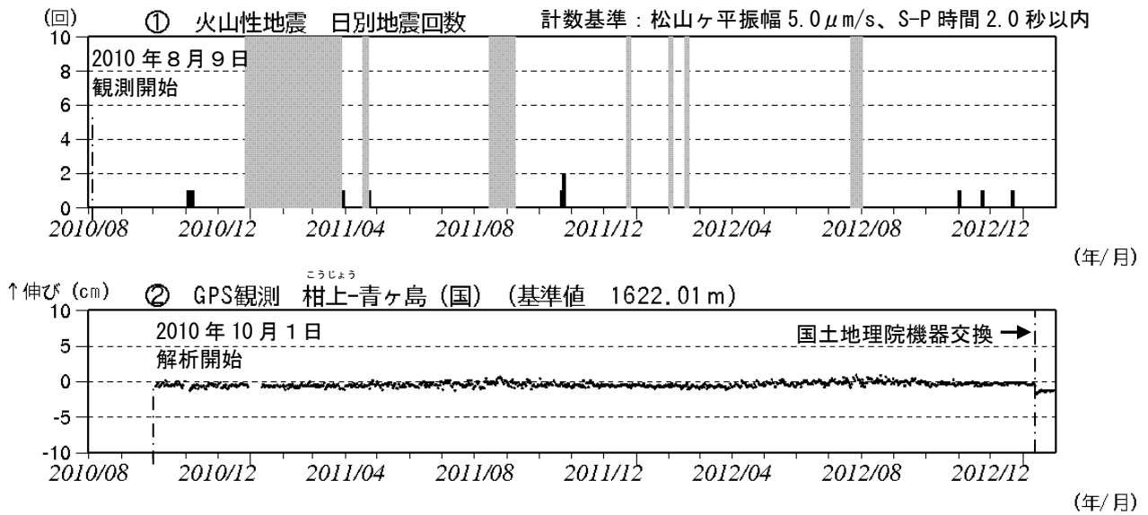
図 2※ 青ヶ島 火山活動の推移 (2010 年 8 月 9 日～2013 年 1 月 31 日)
