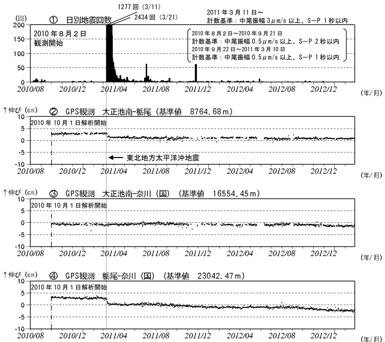
図 3※ 焼岳 火山活動経過図 (2010 年 8 月 2 日～2013 年 2 月 28 日)
