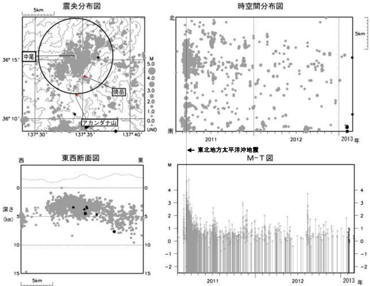
図 4※ 焼岳 広域地震観測網による山体・周辺の地震活動（2011 年 2 月 1 日～2013 年 2 月 28 日）
