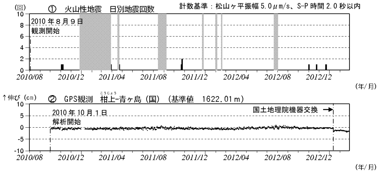
図 2※ 青ヶ島 火山活動の推移 (2010 年 8 月 9 日～2013 年 2 月 28 日)
