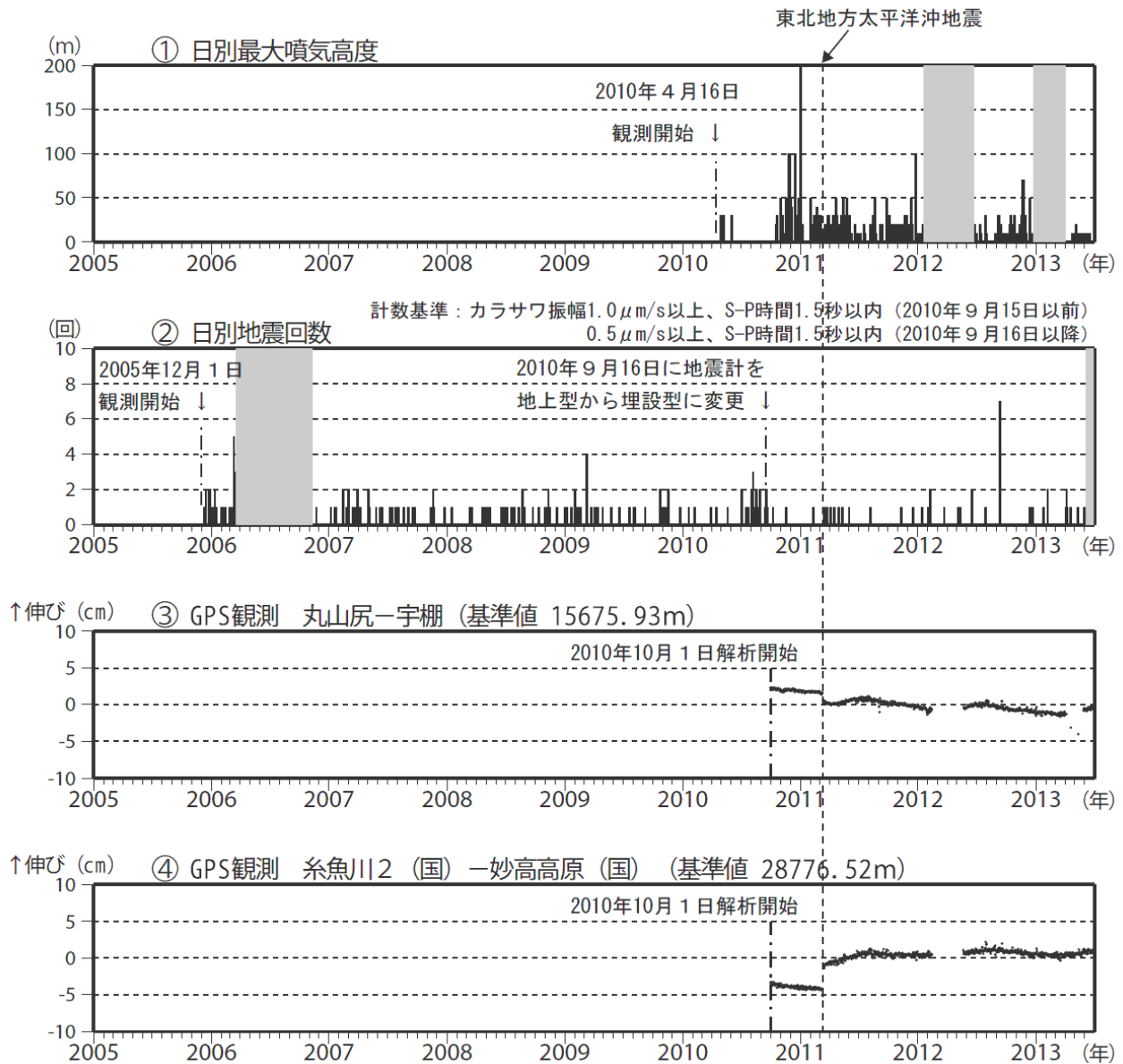
図3 新潟焼山 火山活動経過図（2005年12月1日～2013年6月30日）
