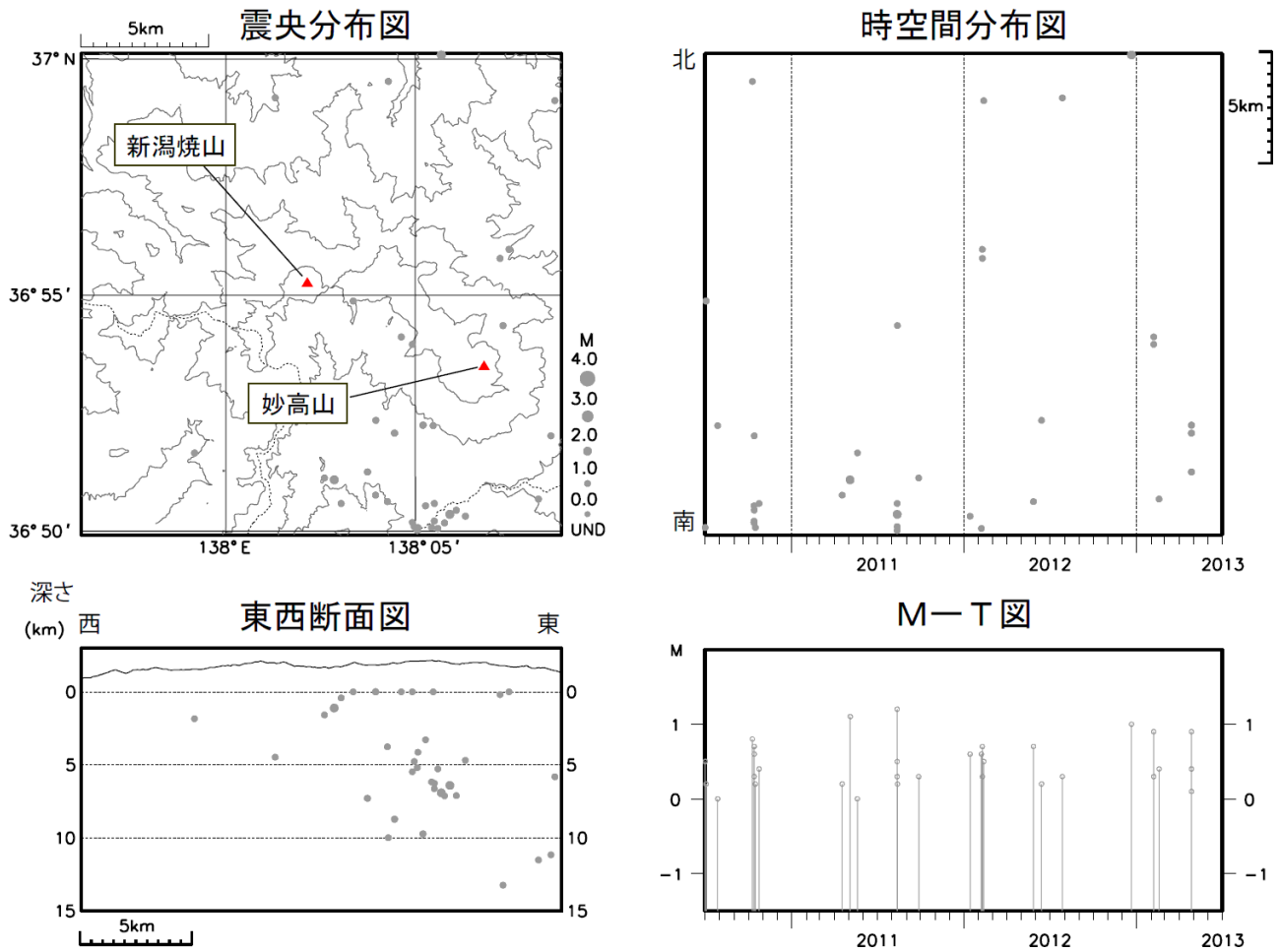
図 4 新潟焼山 広域地震観測網による山体・周辺の地震活動（2010 年 6 月 1 日～2013 年 6 月 30 日）
