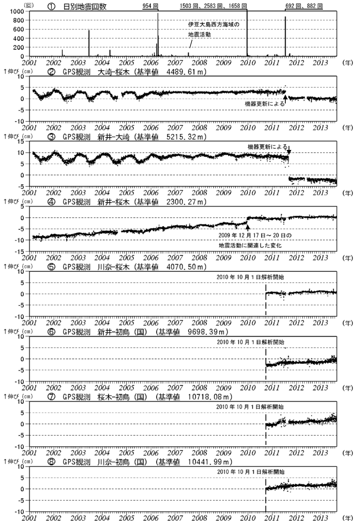
図3 伊豆東部火山群 最近の火山活動経過図（2001年1月～2013年8月）
