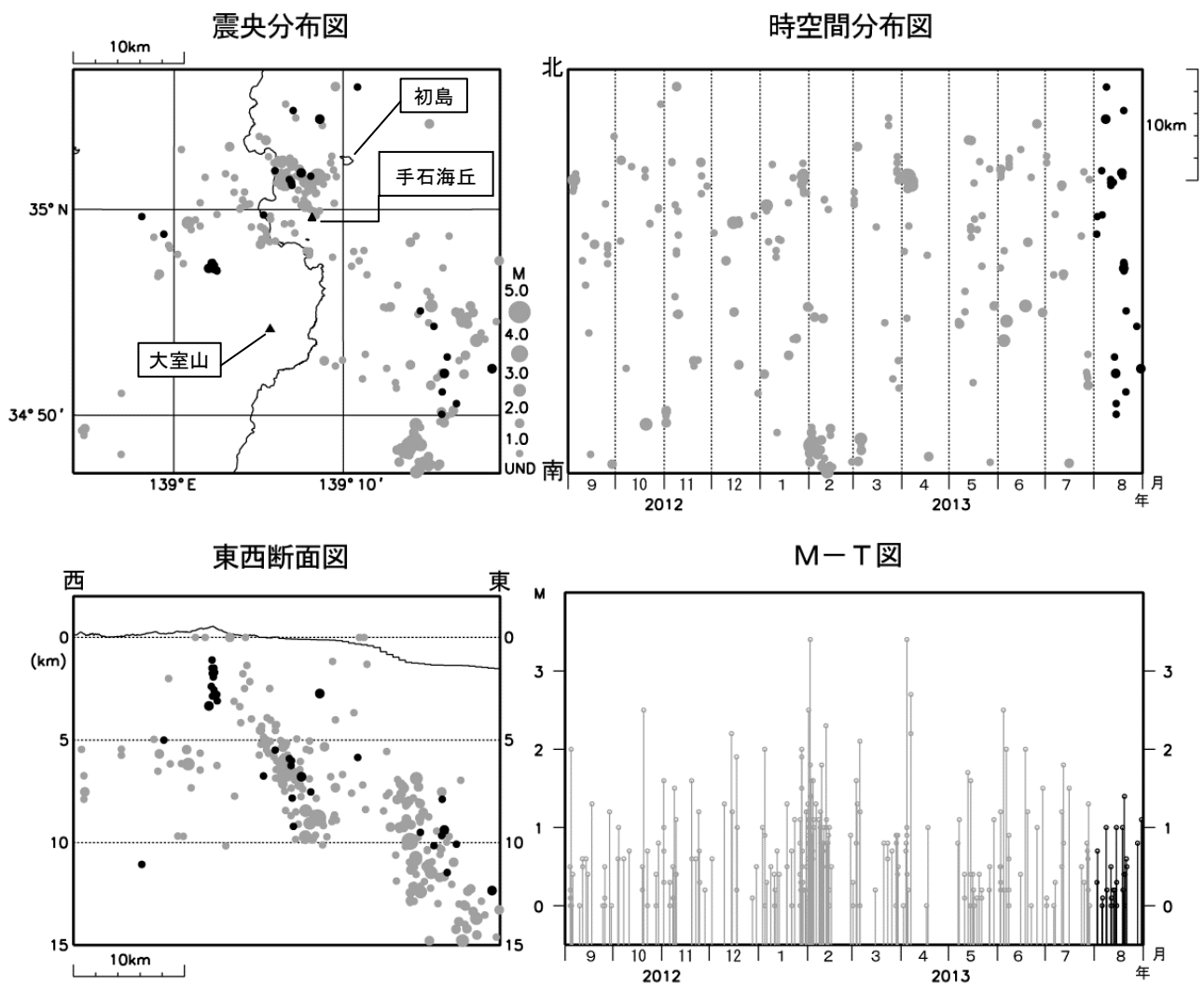
図 2 伊豆東部火山群 広域地震観測網による震源分布図（2012年9月1日～2013年8月31日）
