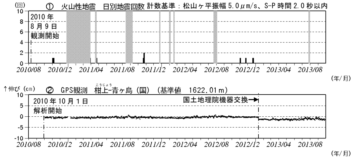
図 2 青ヶ島 火山活動の推移（2010 年 8 月 9 日～2013 年 9 月 30 日）
