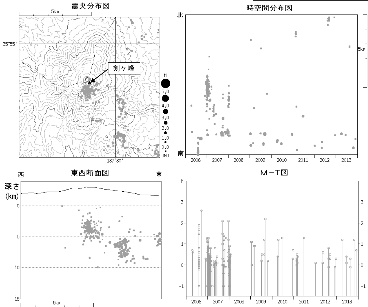
図 4 御嶽山 広域地震観測網による山体・周辺の震源分布図（2006 年 1 月 1 日～2013 年 12 月 31 日） ●：2006 年 1 月 1 日～2013 年 11 月 30 日 ●：2013 年 12 月 1 日～12 月 31 日 M（マグニチュード）は地震の規模を表します。 今期間、震源が決定された地震はありません。 図中の震源要素は一部暫定値が含まれており、後日変更することがあります。
