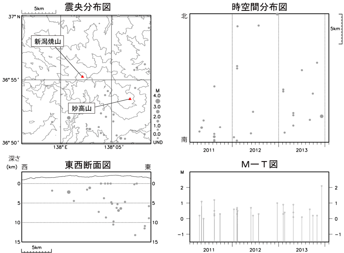
図 4 新潟焼山 広域地震観測網による山体・周辺の地震活動（2011 年 2 月 1 日～2014 年 1 月 31 日）
