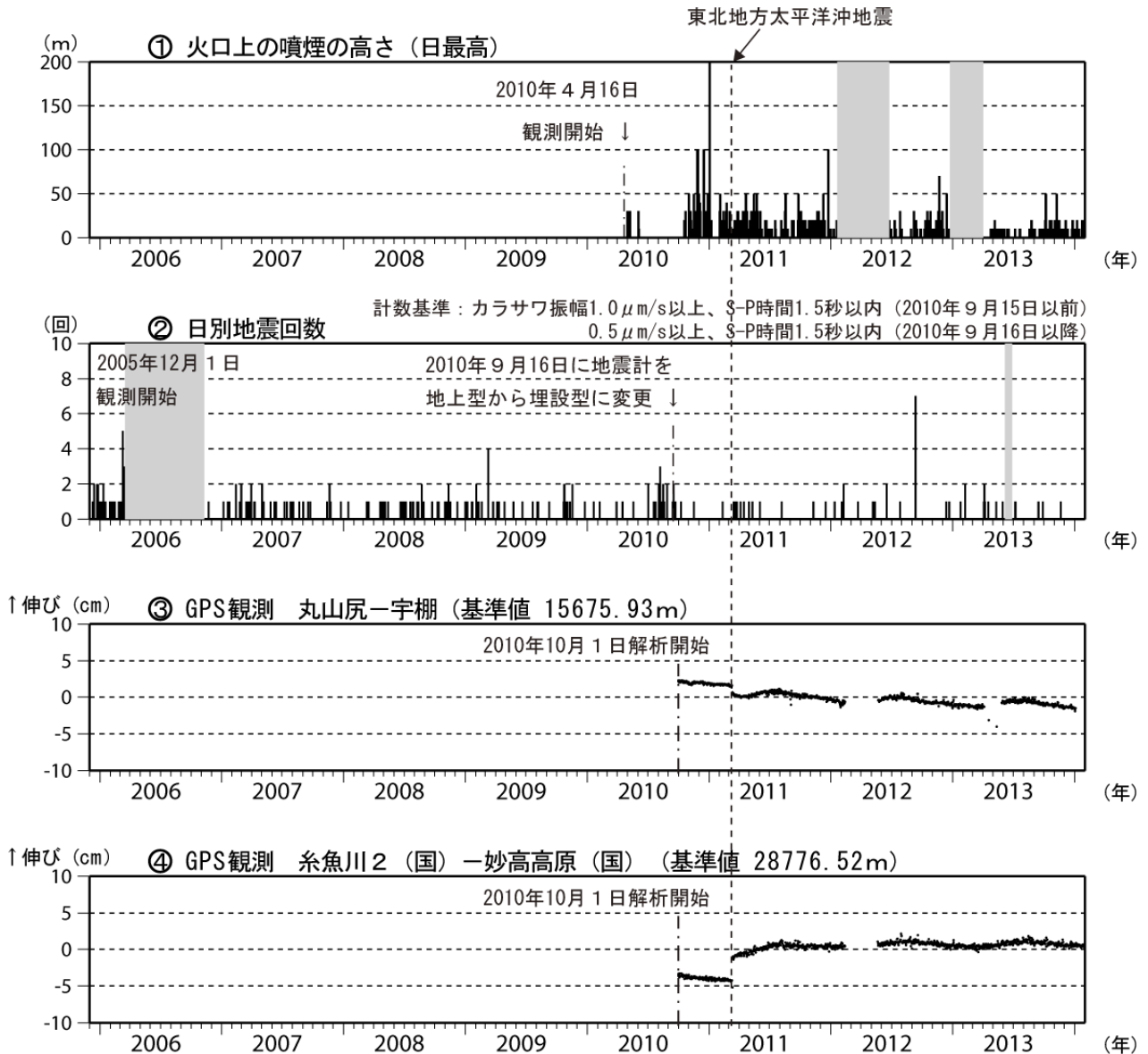
図3 新潟焼山 火山活動経過図（2005年12月1日～2014年1月31日）
