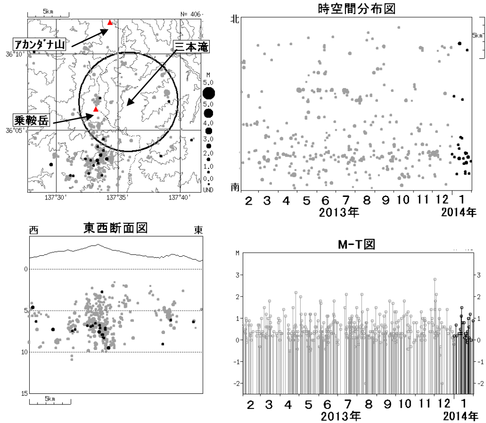
図 3 乗鞍岳 広域地震観測網による山体・周辺の地震活動（2013 年 2 月 1 日～2014 年 1 月 31 日）
