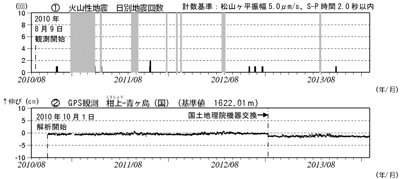
図 2 青ヶ島 火山活動の推移 (2010 年 8 月 9 日～2014 年 1 月 31 日)
