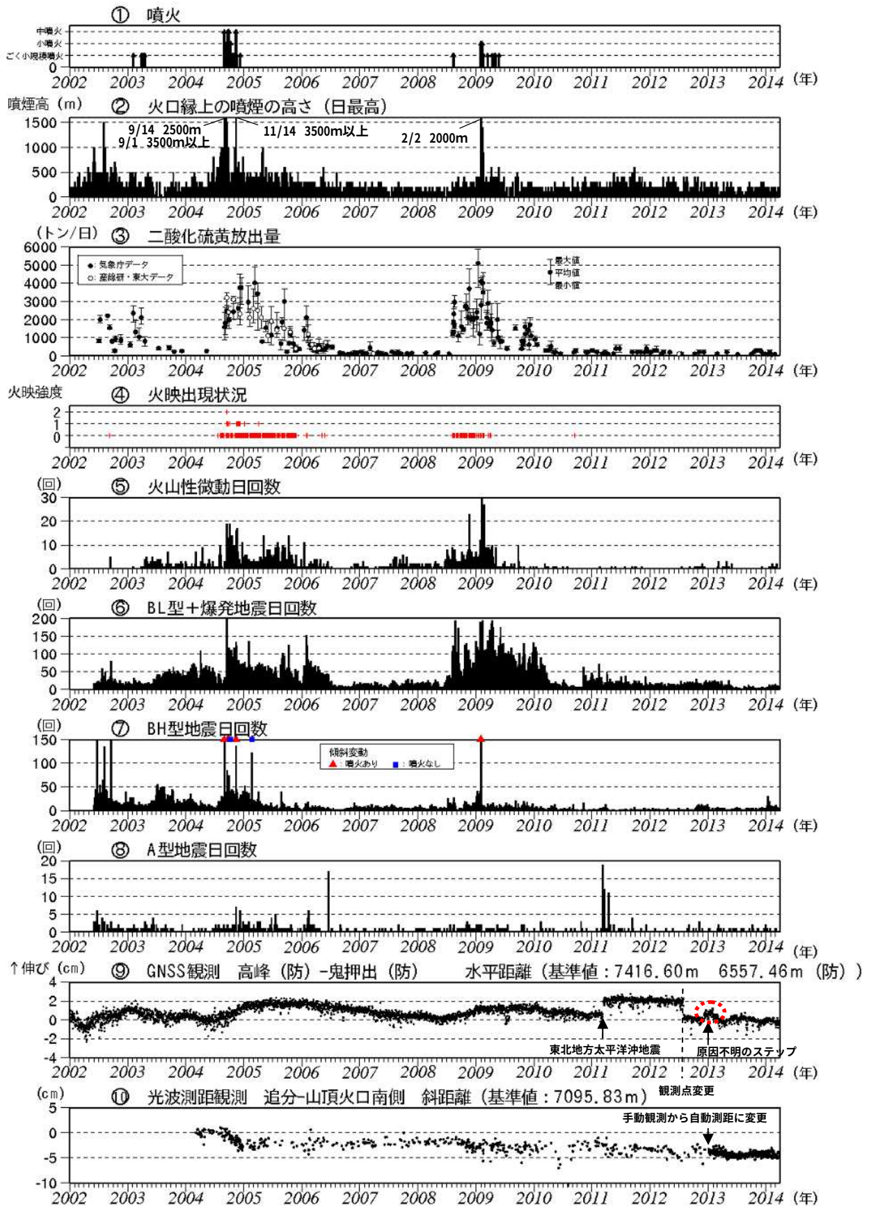
図3 浅間山 最近の火山活動経過図 (2002年1月1日～2014年3月31日)
