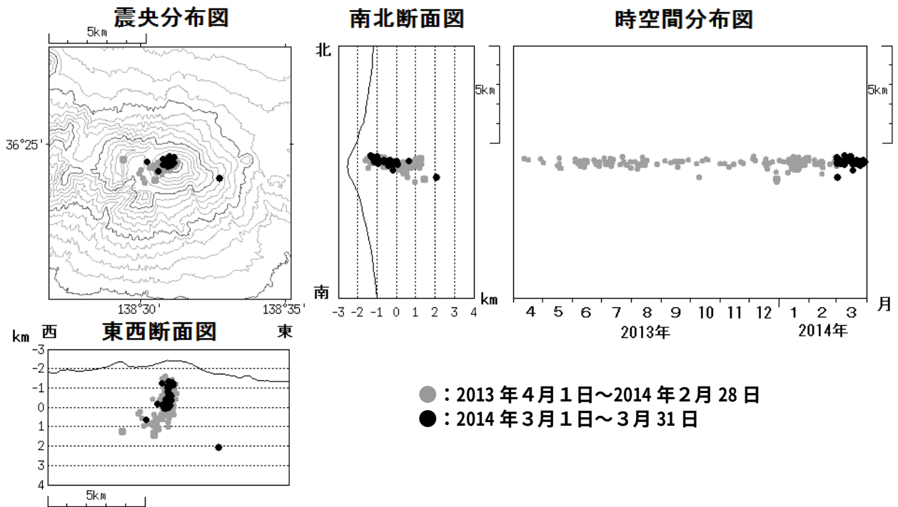
図 4 浅間山 震源分布図（2013 年 4 月 1 日～2014 年 3 月 31 日）
