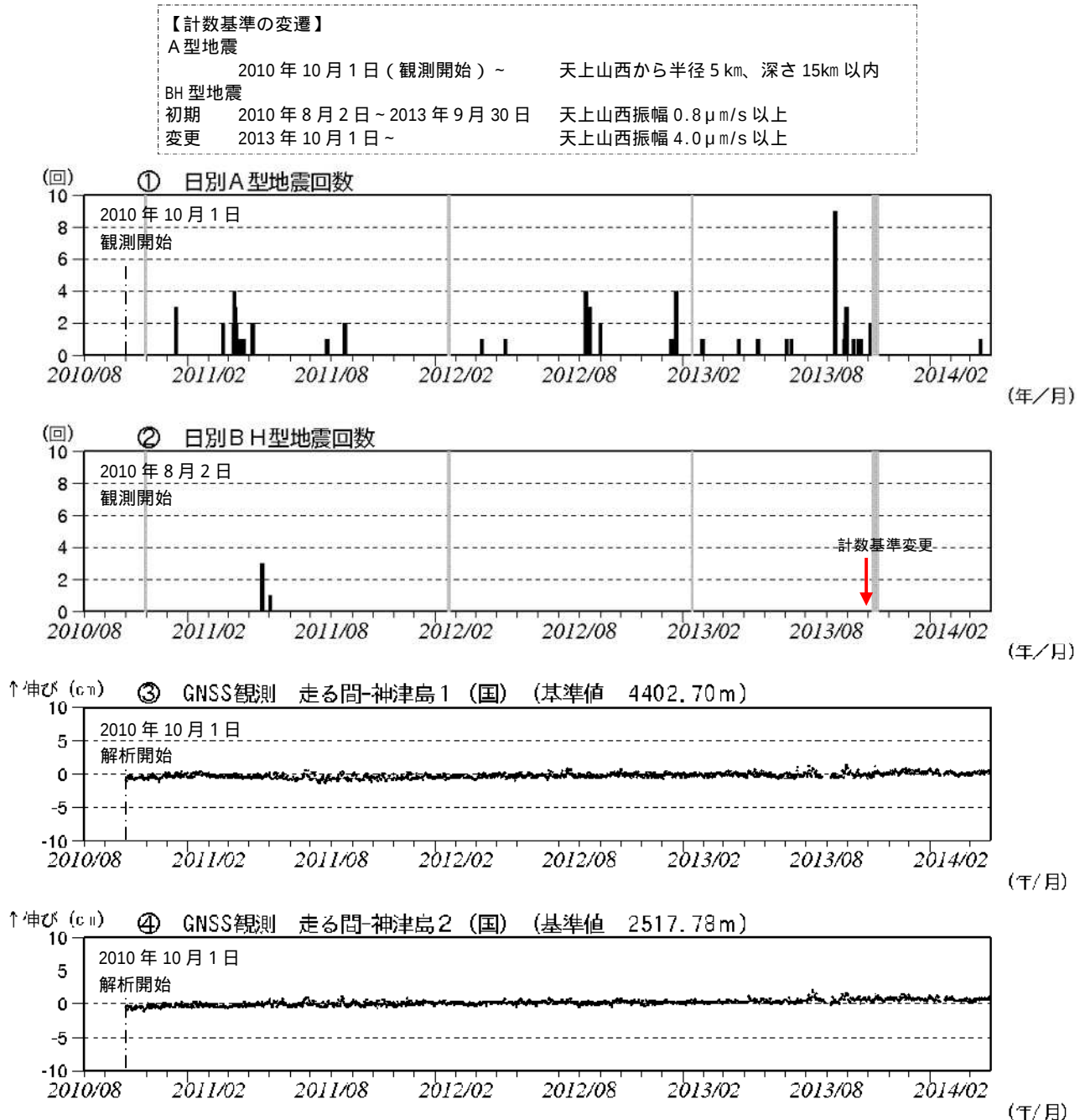
図3 神津島 火山活動経過図(2010年8月2日～2014年3月31日)
