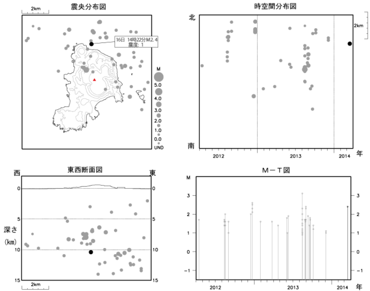
図4 神津島 広域地震観測網による山体・周辺の地震活動（2012 年 4 月 1 日～2014 年 3 月 31 日）
