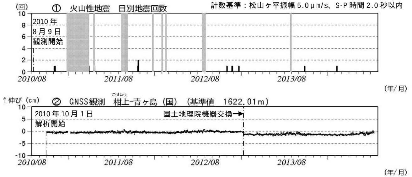
図 2 青ヶ島 火山活動経過図（2010 年 8 月 9 日～2014 年 7 月 31 日）
