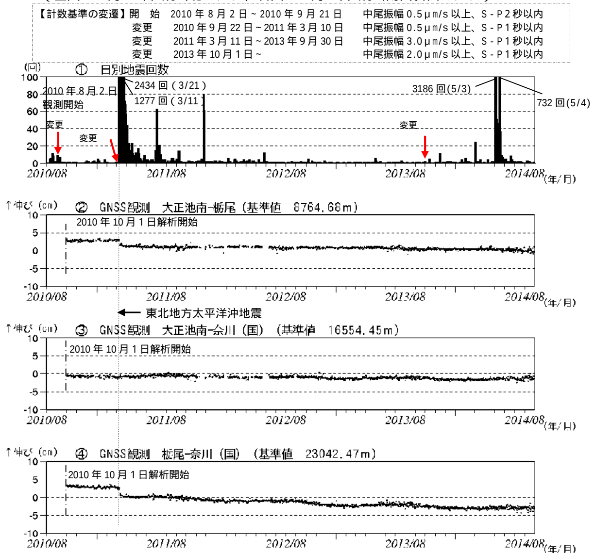
図 3 焼岳 火山活動経過図 (2010年 8 月 2 日 ~ 2014年 8 月 31 日)
