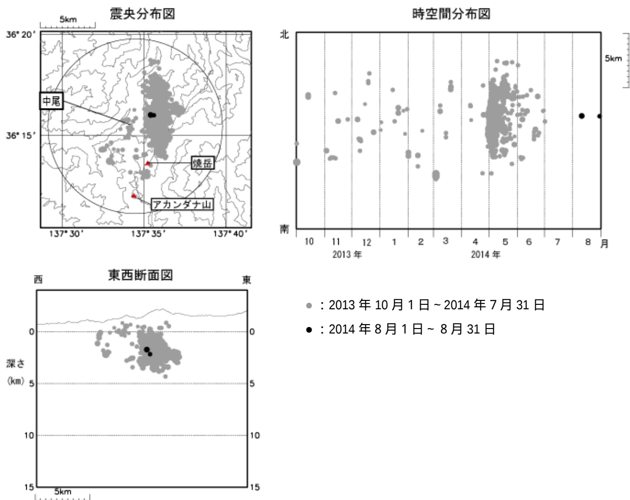
図 4 焼岳 震源分布図（2013 年 10 月 1 日～2014 年 8 月 31 日） 震央分布図中の円は図 3 - の計数対象地震（中尾で S - P 時間 1 秒以内）のおよその範囲を示します。
