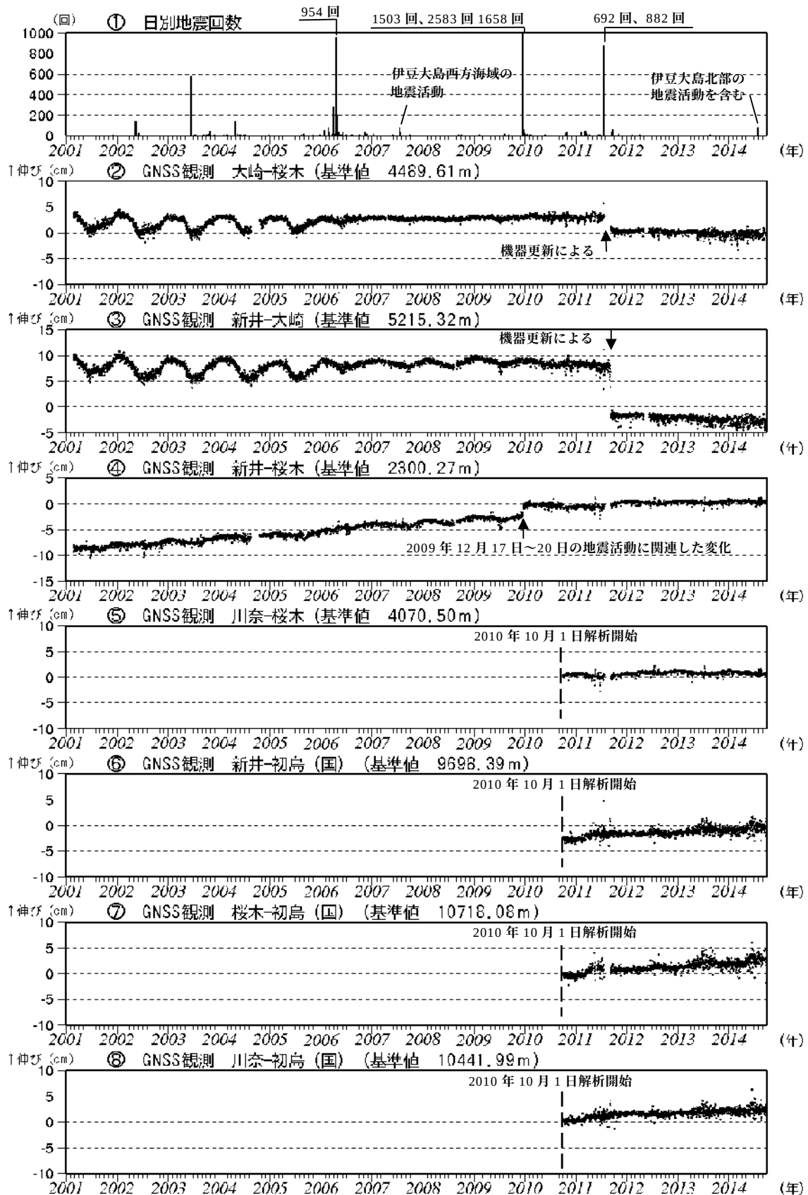
図3 伊豆東部火山群 火山活動経過図（2001年1月～2014年9月）
