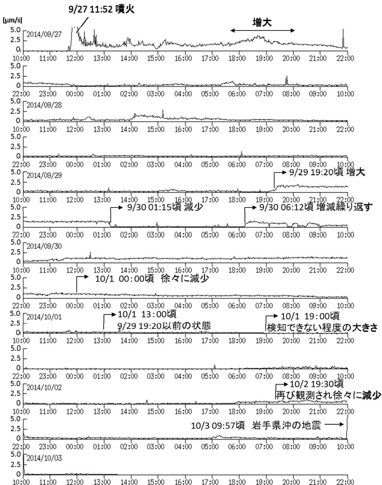
図1 御嶽山 田ノ原上観測点（剣ヶ峰南東約2 km）の上下動地震波形の1分間振幅平均値の推移 （2014年9月27日10時～10月3日13時30分）
