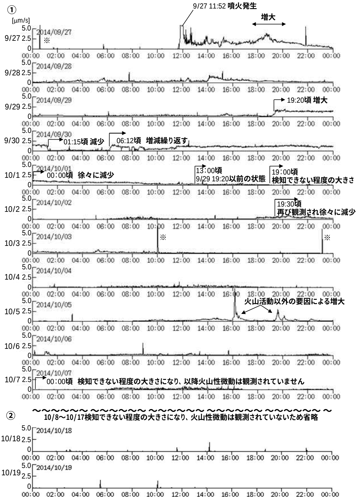
図 4 御嶽山 田の原上観測点（剣ヶ峰の南東約 2 km）の上下動地震波形の 1 分間振幅平均値の推移
