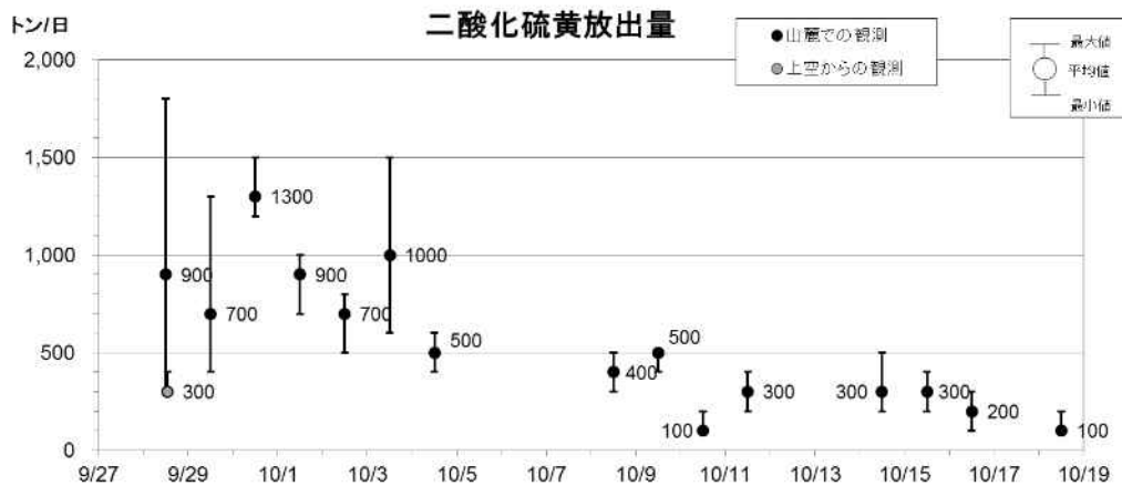
図2 御嶽山 火山ガス（二酸化硫黄）観測結果（9月28日～10月18日）
