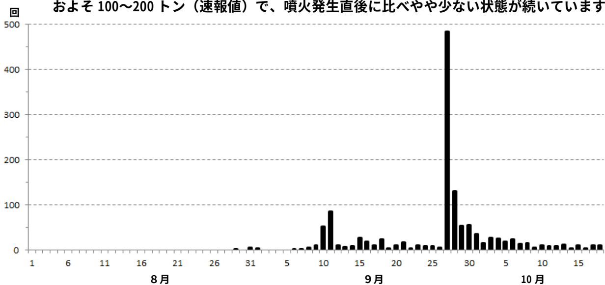
図3 御嶽山 日別地震回数（2014年8月1日～10月18日（速報値含む））
