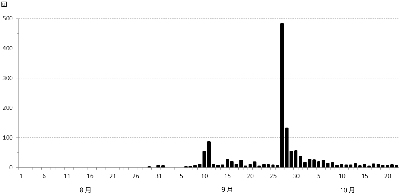
図 2 御嶽山 日別地震回数（2014 年 8 月 1 日～10 月 22 日（速報値含む）） ・火山性地震は、噴火発生直後に比べて減少し、やや少ない状態で推移しています。
