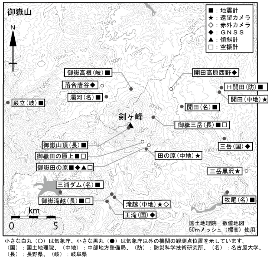
図 1 御嶽山 観測点配置図
