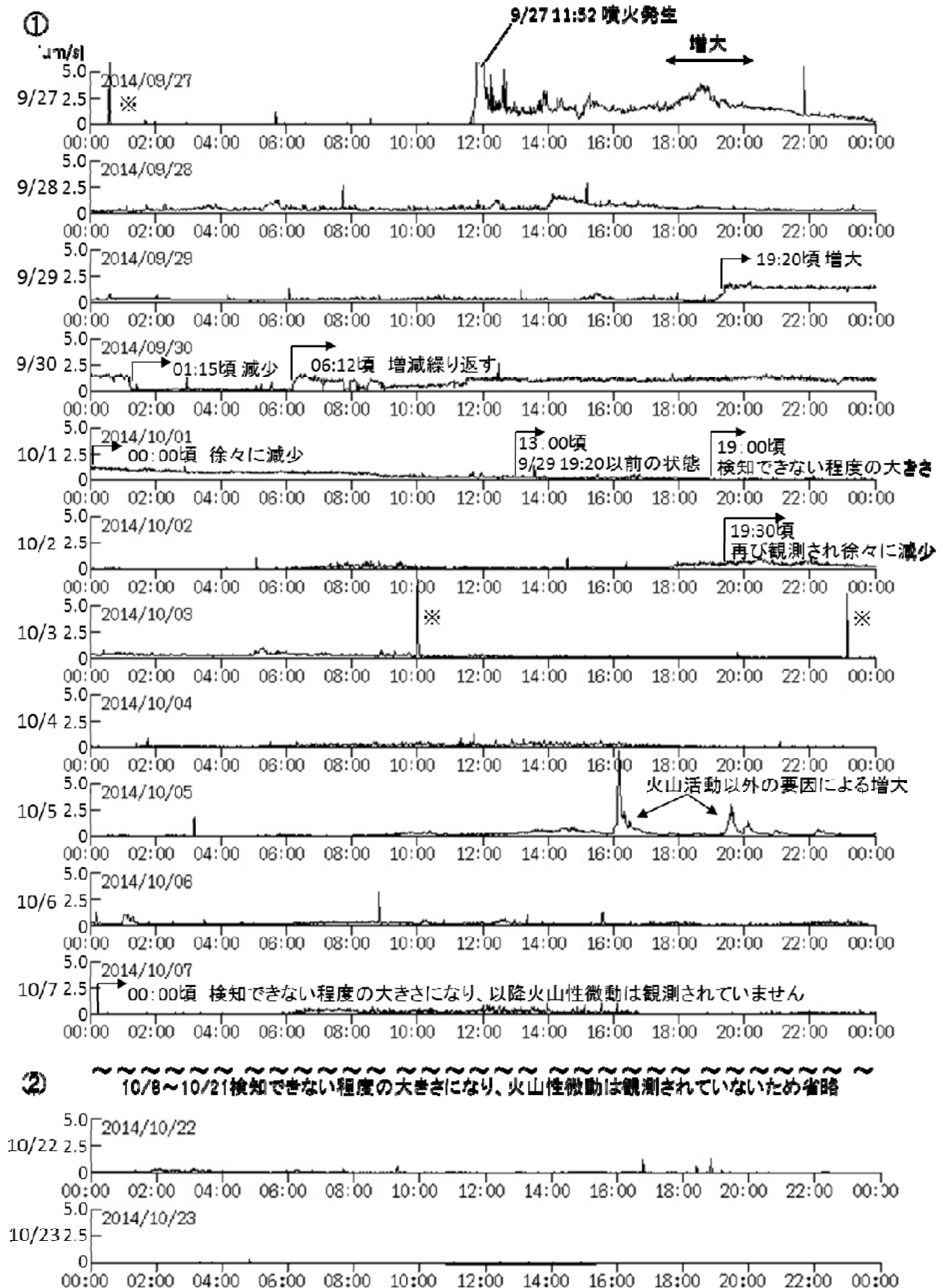
図3 御嶽山 田の原上観測点（剣ヶ峰の南東約2km）の上下動地震波形の1分間振幅平均値の推移 期間 2014年9月27日00時～10月7日24時00分 期間 2014年10月22日00時～10月23日15時20分 火山活動以外の地震による ・火山性微動は、検知できない大きさになった10月7日以降は観測されていません。
