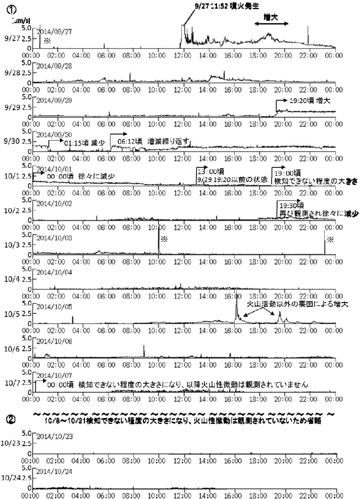
図3 御嶽山 田の原上観測点（剣ヶ峰の南東約2 km）の上下動地震波形の1分間振幅平均値の推移 期間 2014年9月27日00時～10月7日24時00分 期間 2014年10月23日00時～10月24日15時20分 火山活動以外の地震による ・火山性微動は、検知できない大きさになった10月7日以降は観測されていません。 御嶽山
