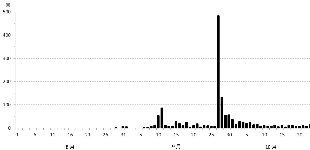
図 2 御嶽山 日別地震回数（2014 年 8 月 1 日～10 月 23 日（速報値含む））
