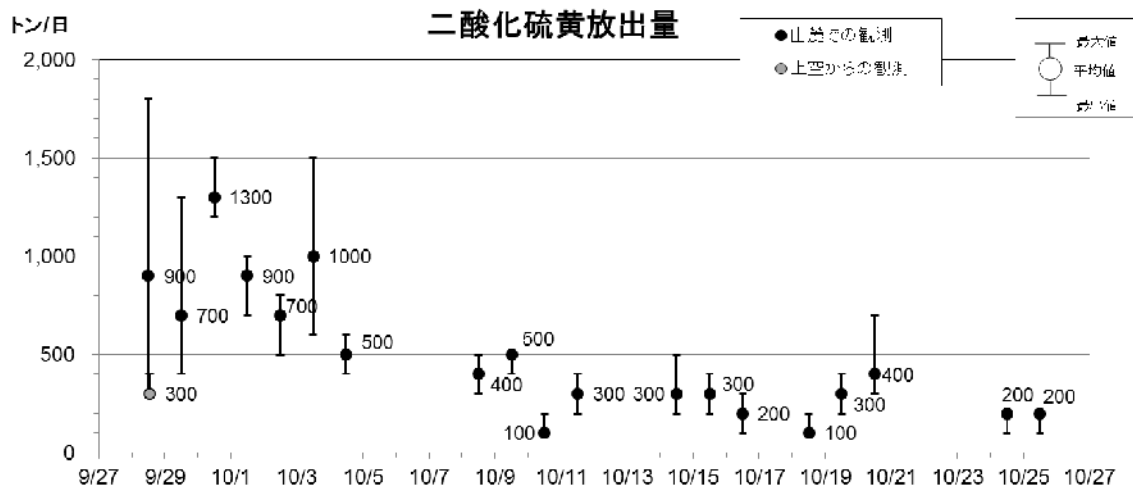
図2 御嶽山 火山ガス（二酸化硫黄）観測結果（9月28日～10月26日）
