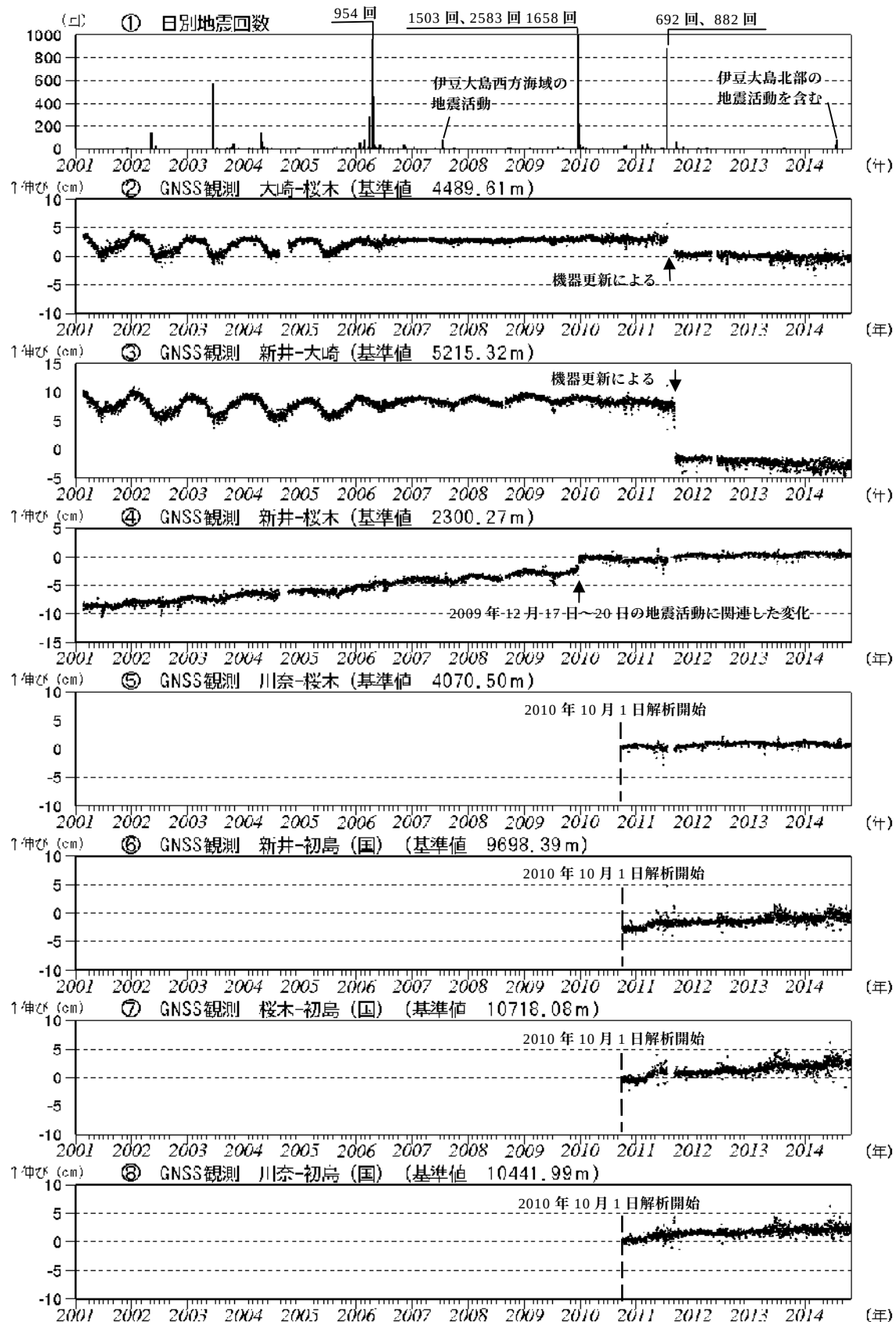
図3 伊豆東部火山群 火山活動経過図 (2001年1月～2014年10月)
